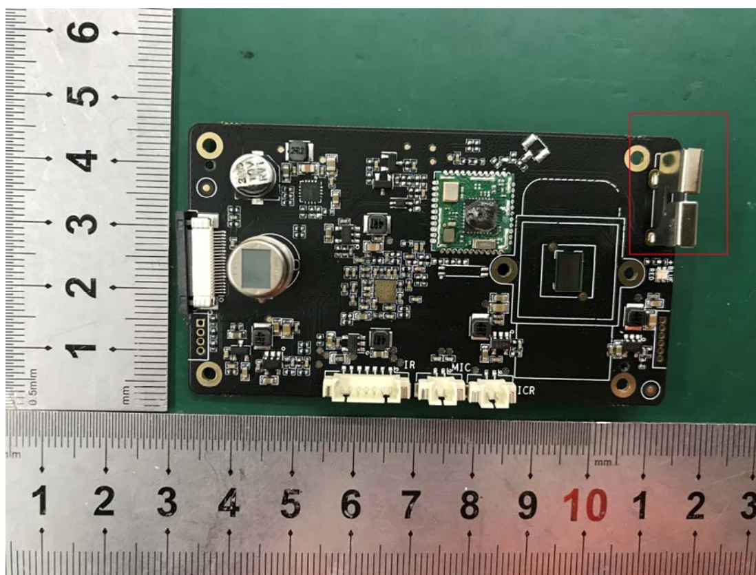
Antenna
