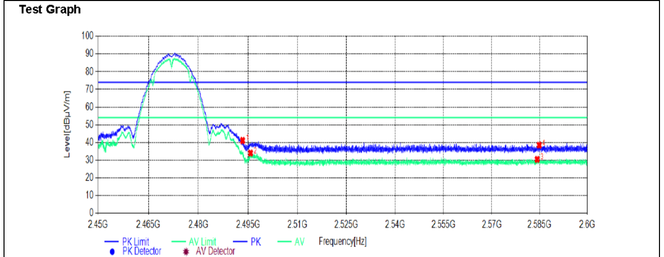
Horizontal (802.11b-2462MHz)
