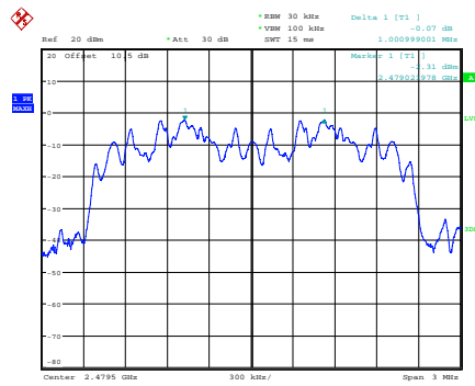
\pi/4 -DQPSK_High
