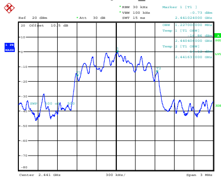
\pi/4 -DQPSK_Middle
