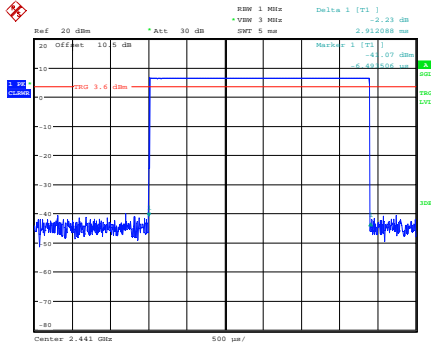
GFSK_Hopping_DH5
