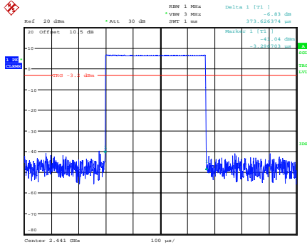
GFSK_Hopping_DH1
