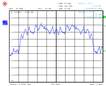
\pi/4 -DQPSK_Low
