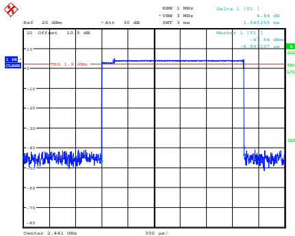
\pi/4 -DQPSK_Hopping_2DH3
