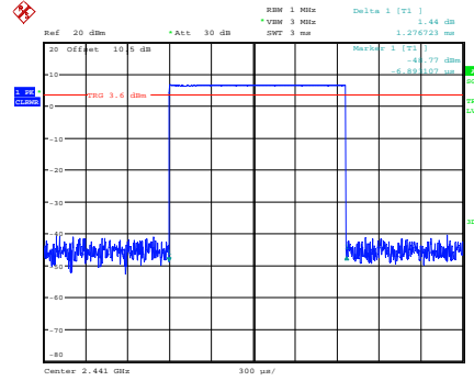
GFSK_Hopping_DH3
