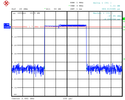
\pi/4 -DQPSK_Hopping_2DH1
