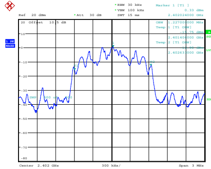
\pi/4 -DQPSK_Low
