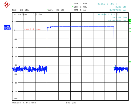
\pi/4 -DQPSK_Hopping_2DH5
