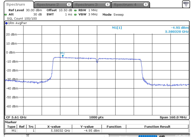
ac80_5610MHz_Chain 0
