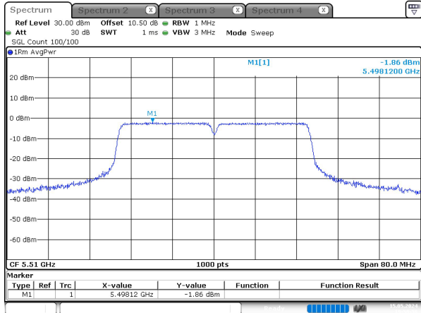
n40_5510MHz_Chain 0
