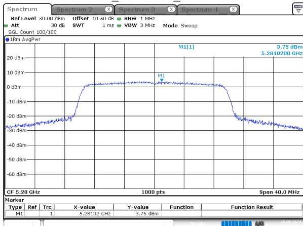
ax20_5280MHz_Chain 0
