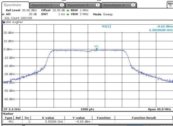
n20_5500MHz_Chain 0
