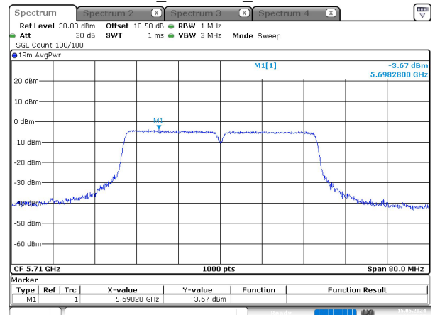
n40_5710MHz_Chain 0
