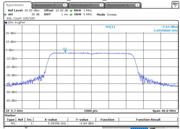
ax20_5700MHz_Chain 0
