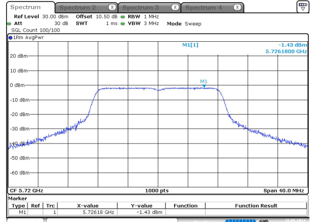
a_5720MHz_Chain 0
