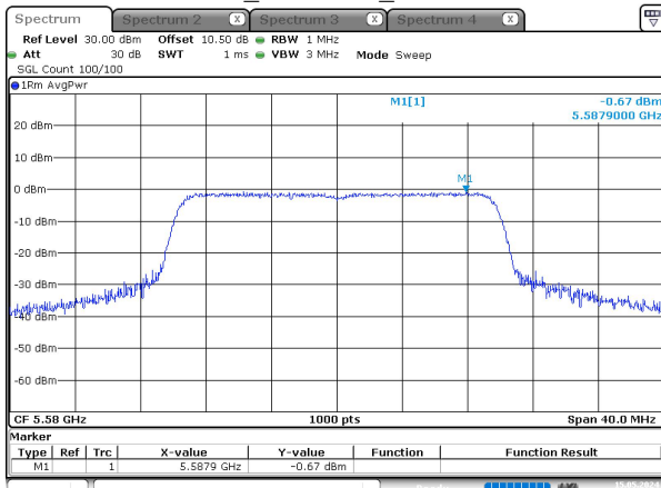
ax20_5580MHz_Chain 0
