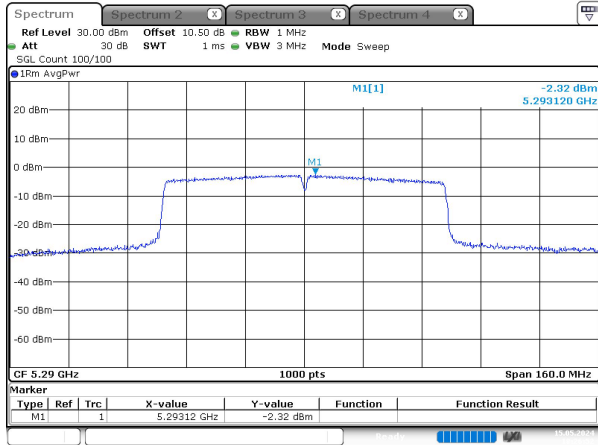
ac80_5290MHz_Chain 0
