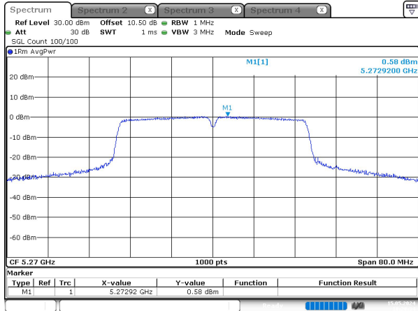
n40_5270MHz_Chain 0
