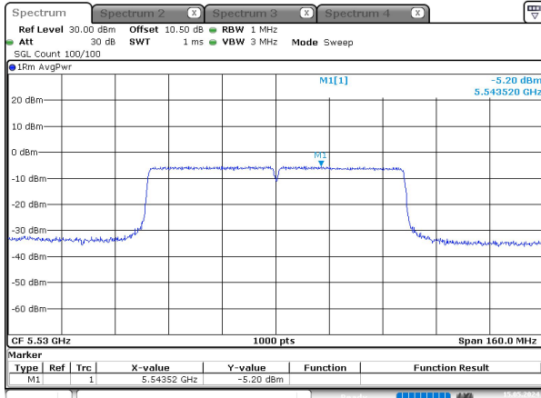
ac80_5530MHz_Chain 0
