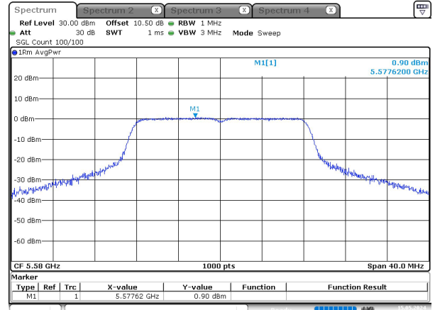
a_5580MHz_Chain 0
