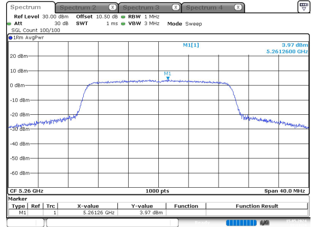
ax20_5260MHz_Chain 0
