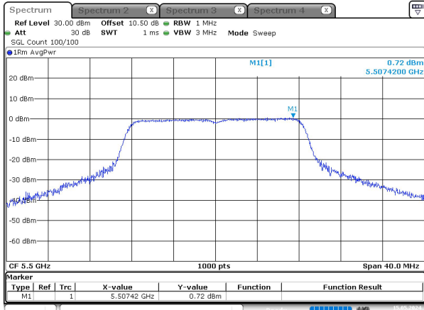
a_5500MHz_Chain 0
