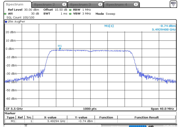
ax20_5500MHz_Chain 0
