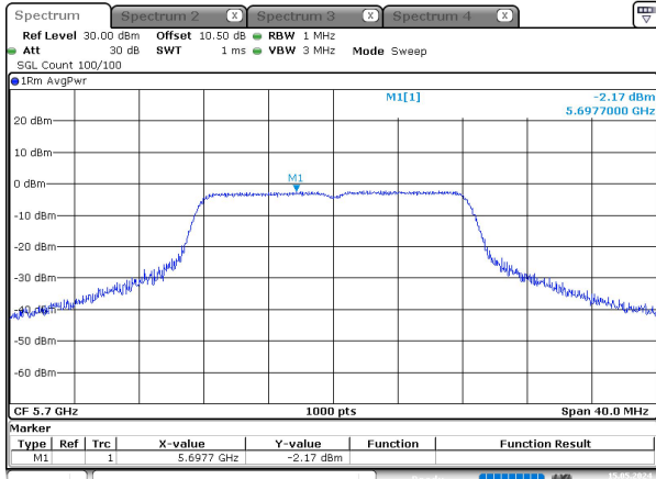
a_5700MHz_Chain 0
