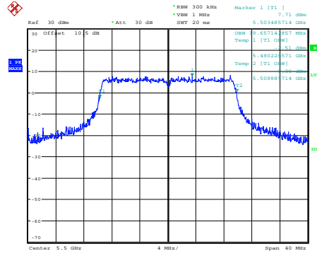
ax20_5500MHz_Chain 0
