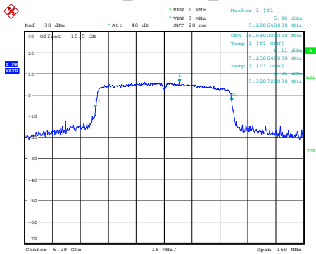
ac80_5290MHz_Chain 0
