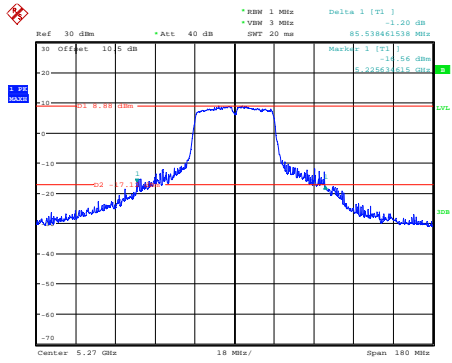
n40_5270MHz_Chain 0
