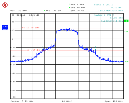
ac80_5290MHz_Chain 0
