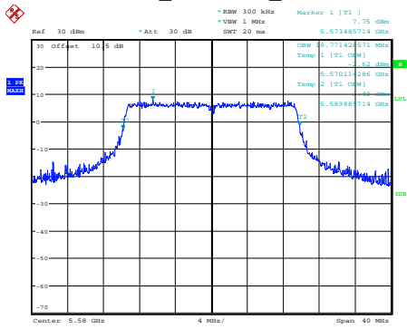
ax20_5580MHz_Chain 0
