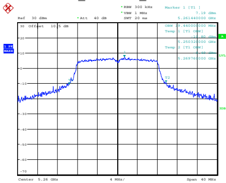
a_5260MHz_Chain 0
