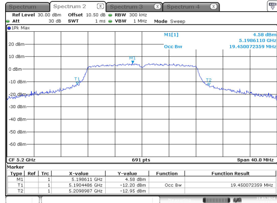
a_5200MHz_Chain 0
