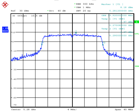
ax20_5280MHz_Chain 0
