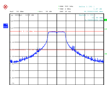
a_5720MHz_Chain 0
