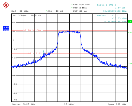
ax20_5260MHz_Chain 0
