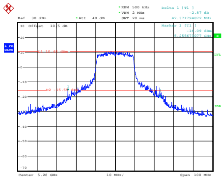
ax20_5280MHz_Chain 0
