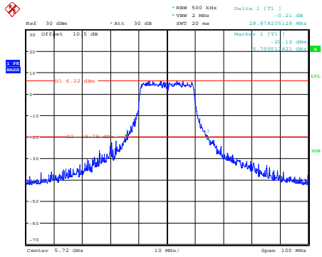
ax20_5720MHz_Chain 0
