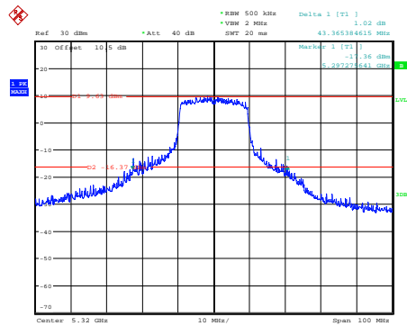
ax20_5320MHz_Chain 0
