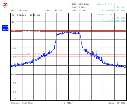
ax20_5200MHz_Chain 0
