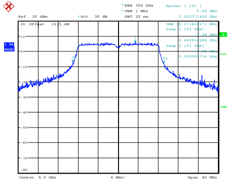
a_5500MHz_Chain 0
