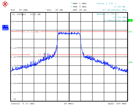
ax40_5710MHz_Chain 0
