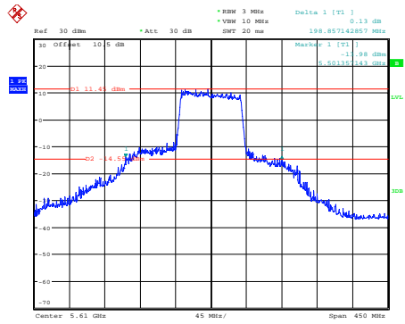
ax80_5610MHz_Chain 0
