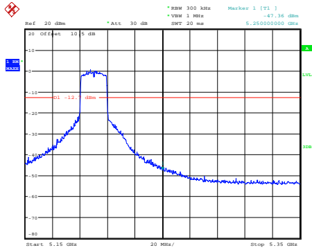
ax20_5200MHz_Chain 0
