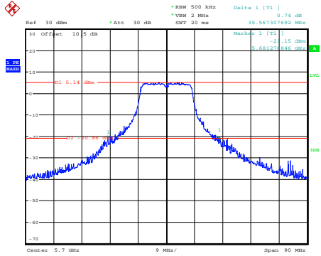
a_5700MHz_Chain 0
