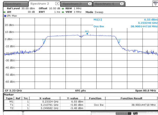
n40_5230MHz_Chain 0
