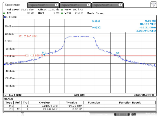
n20_ 5240MHz_Chain 0
