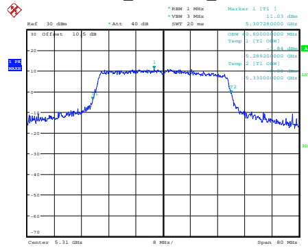
ax40_5310MHz_Chain 0
