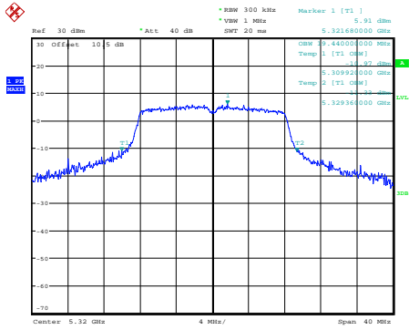
a_5320MHz_Chain 0
