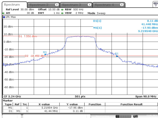
a_ 5240MHz_Chain 0
