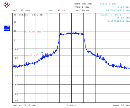
ax20_5180MHz_Chain 0
