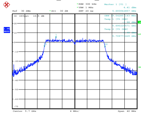
ax20_5700MHz_Chain 0
