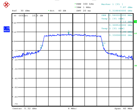
ax20_5320MHz_Chain 0
