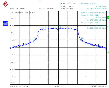
a_5280MHz_Chain 0
