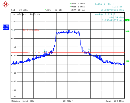
ax40_5190MHz_Chain 0
