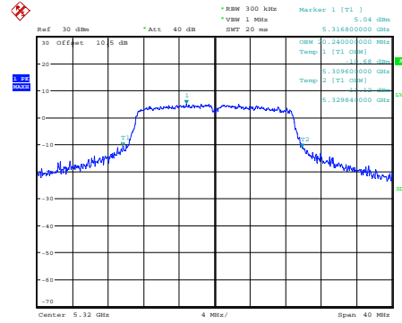
n20_5320MHz_Chain 0
