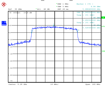
ax80_5290MHz_Chain 0
