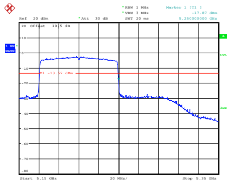
ax80_5210MHz_Chain 0
