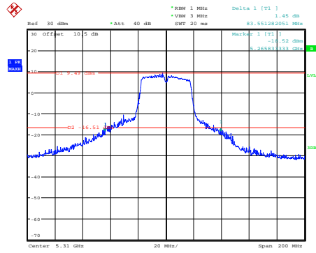
n40_5310MHz_Chain 0
