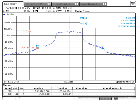
n20_ 5180MHz_Chain 0
