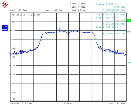
n40_5270MHz_Chain 0
