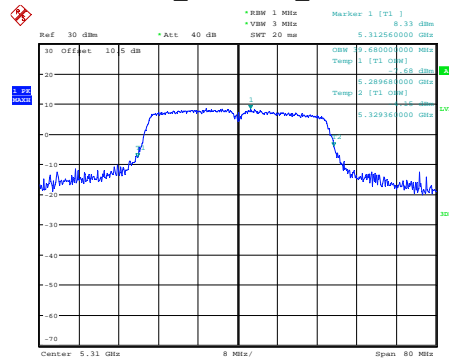
n40_5310MHz_Chain 0
