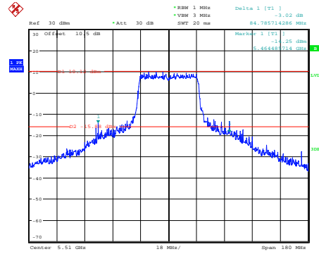
ax40_5510MHz_Chain 0
