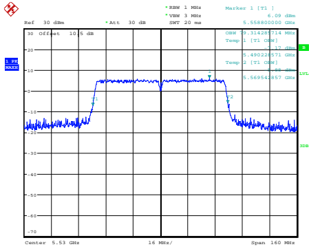
ac80_5530MHz_Chain 0
