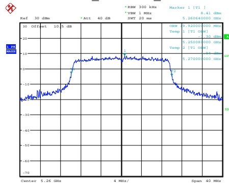
ax20_5260MHz_Chain 0
