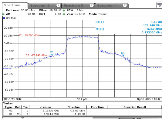
ax80_5210MHz_Chain 0
