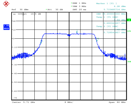
n40_5710MHz_Chain 0
