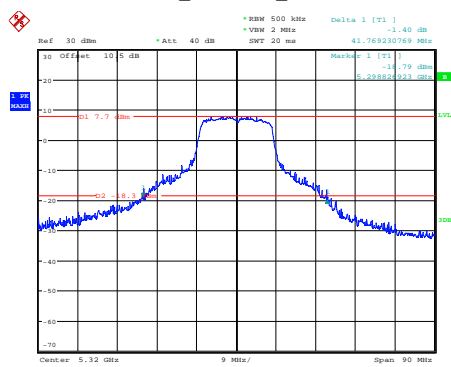
a_5320MHz_Chain 0
