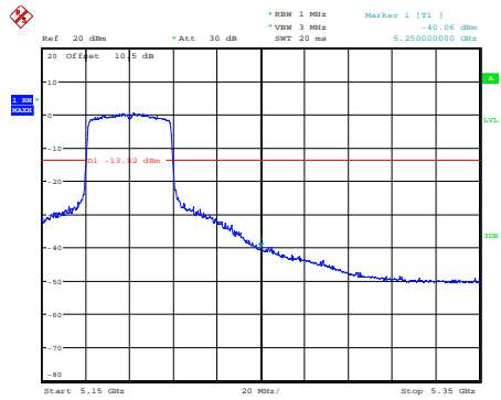
ax40_5190MHz_Chain 0
