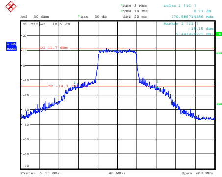
ax80_5530MHz_Chain 0
