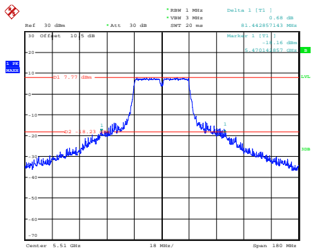
n40_5510MHz_Chain 0
