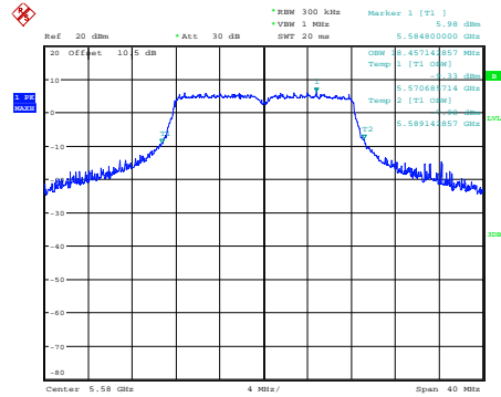
a_5580MHz_Chain 0
