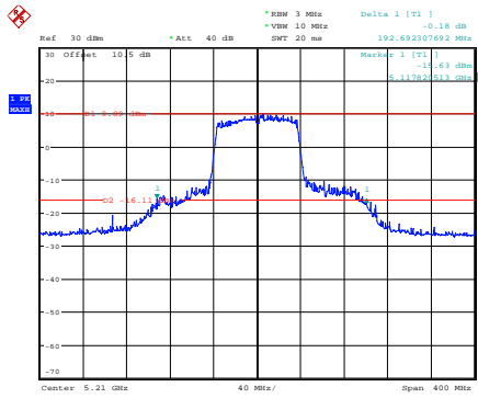
ac80_5210MHz_Chain 0
