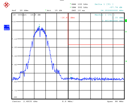
b_2462MHz
