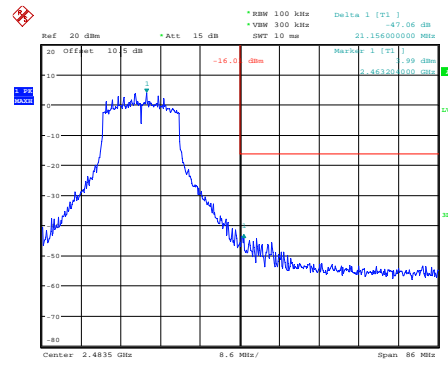
g_2462MHz
