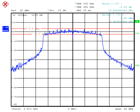
ax20_2412MHz
