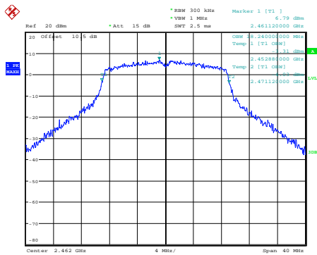
n20_2462MHz
