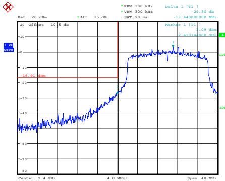
ax20_2412MHz
