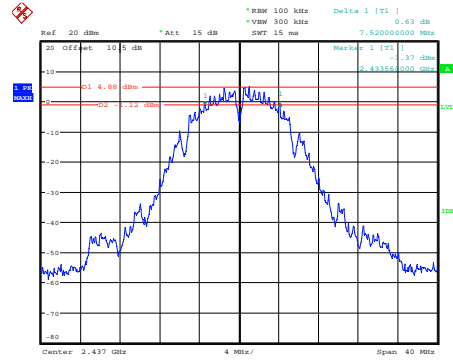
b_2437MHz
