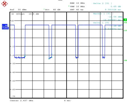
b_2437MHz
