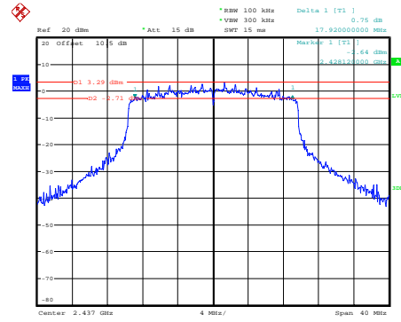
ax20_2437MHz
