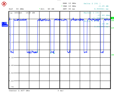
ax20_2437MHz
