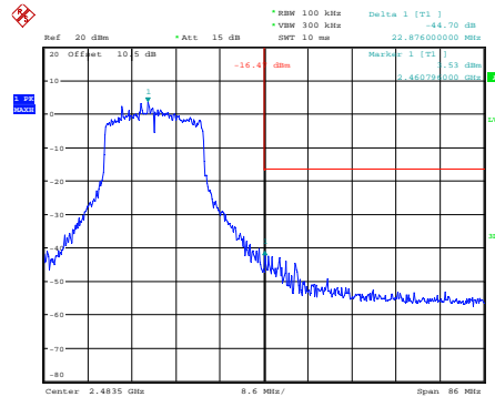
ax20_2462MHz
