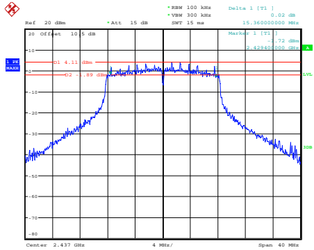
g_2437MHz
