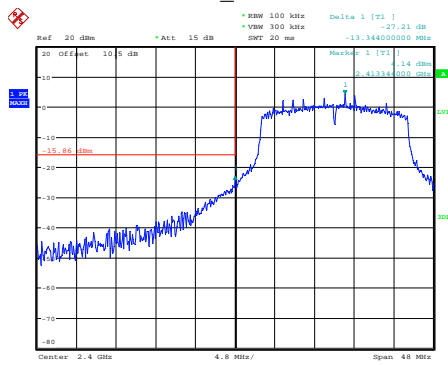
n20_2412MHz
