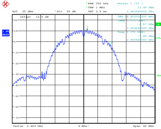
b_2462MHz
