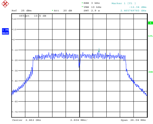
n20_2462MHz
