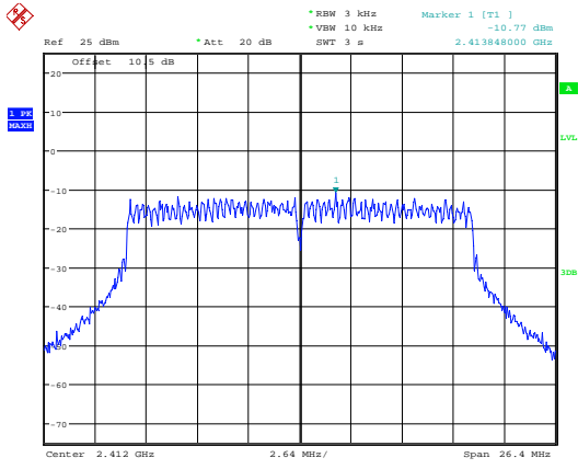
n20_2412MHz
