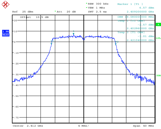
n20_2412MHz
