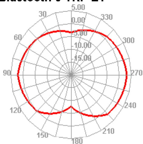
Bluetooth 0 TRP E1
