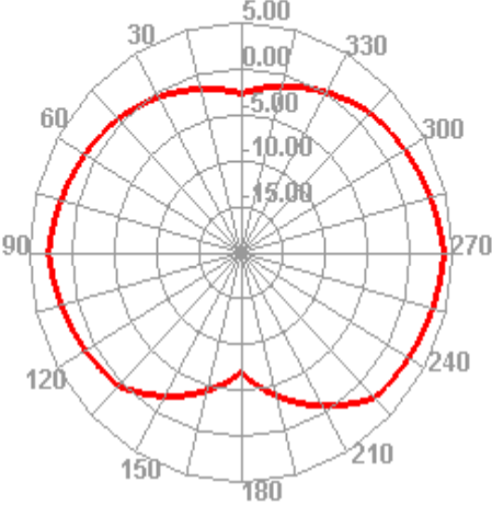
Bluetooth 39 TRP E1
