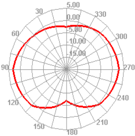
Bluetooth 39 TRP E2
