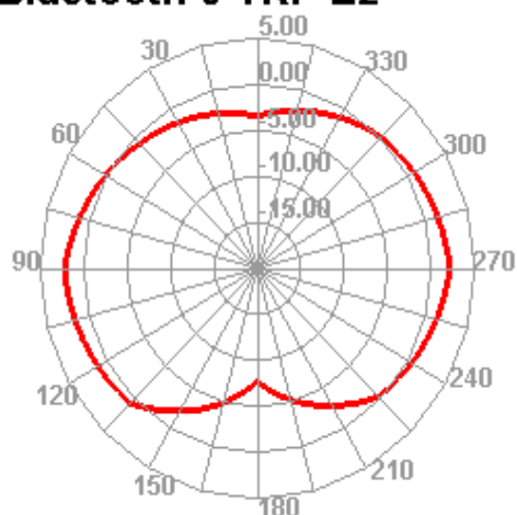
Bluetooth 0 TRP E2
