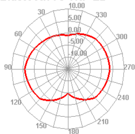
Bluetooth 78 TRP E2
