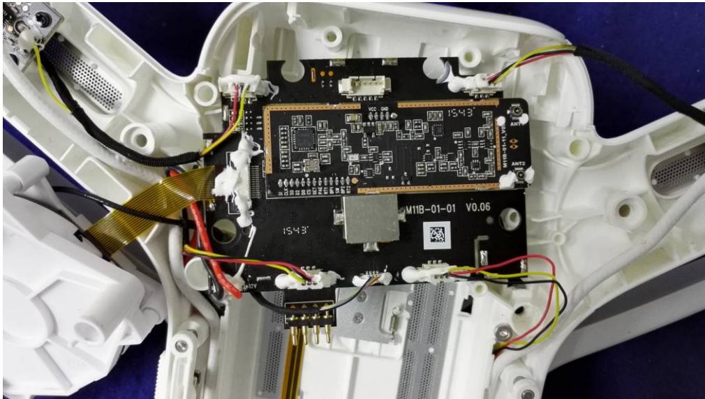
(3) EUT Photo
