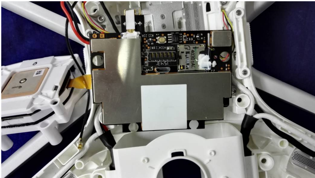
(4) EUT Photo
