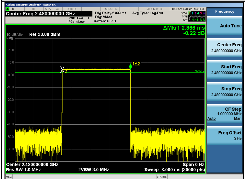
Test_Graph_GFSK_HOP_ANT1_NA_1Mbps_2480_Time per Burst
