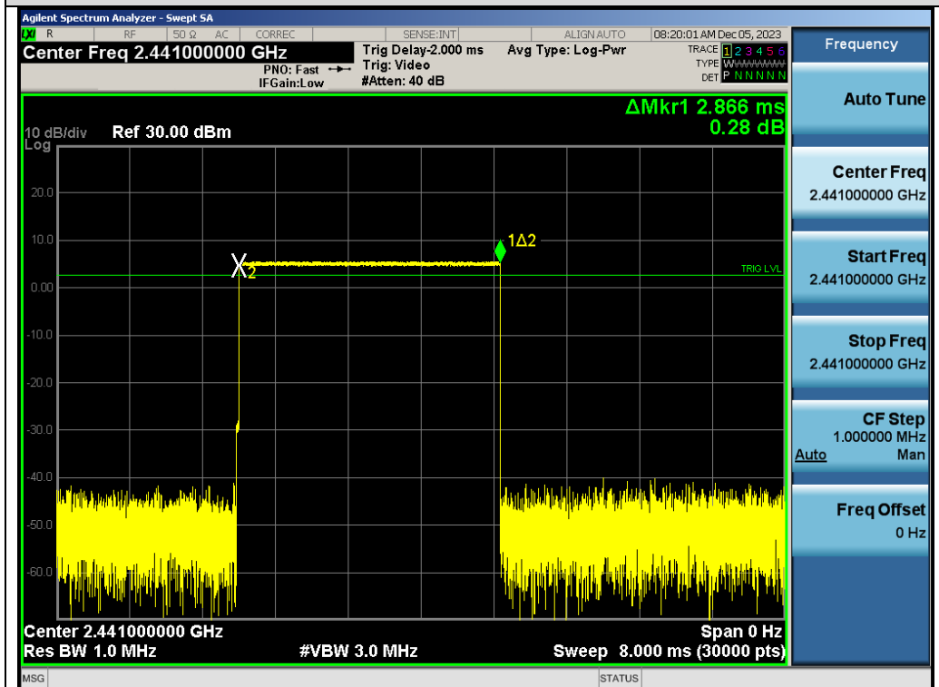
Test_Graph_GFSK_HOP_ANT1_NA_1Mbps_2441_Time per Burst
