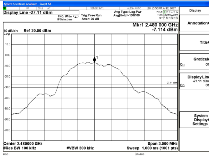
2479 – 2481 MHz
