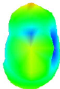
2400.000MHz E1
