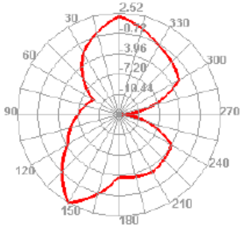
2500.000MHz E1
