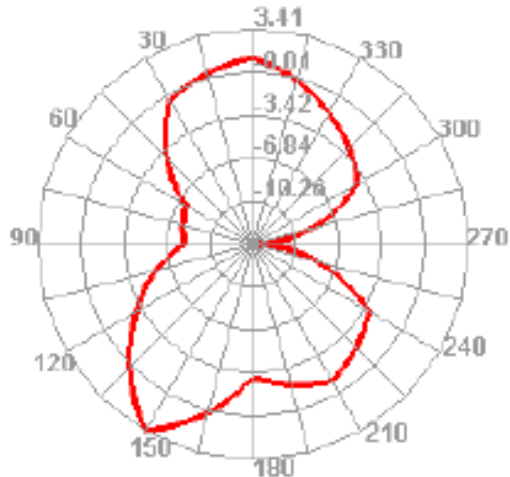
2400.000MHz E1
