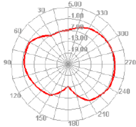
2500.000MHz H
