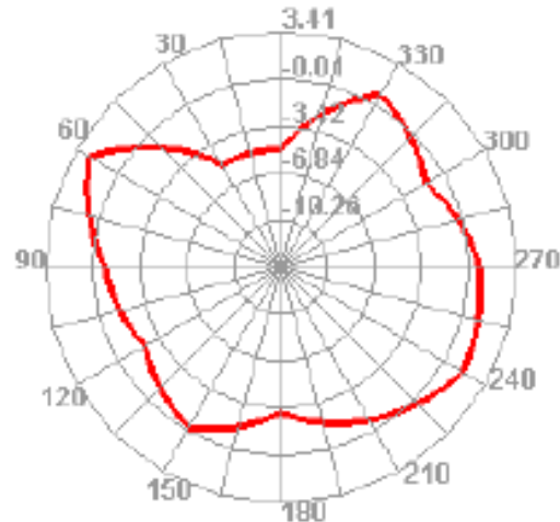
2400.000MHz E2
