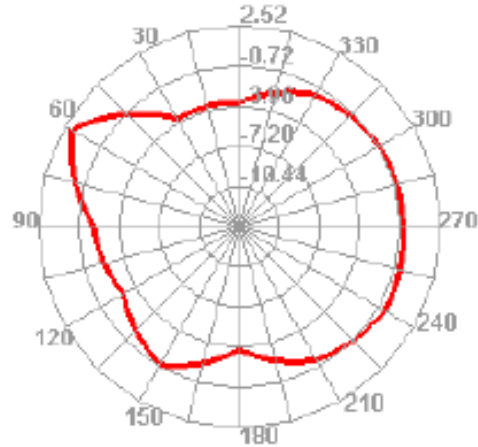
2500.000MHz E2
