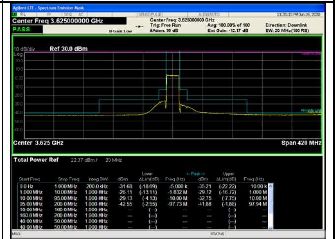
20MHz - Middle CH QPSK
