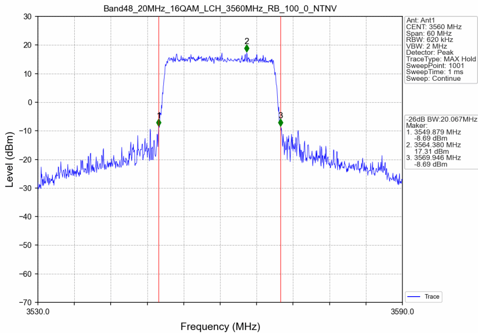
Band48_20MHz_16QAM_LCH_3560MHz_RB_100_0_NTNV
