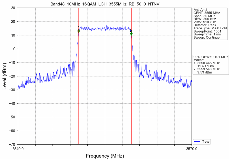
Band48_10MHz_16QAM_LCH_3555MHz_RB_50_0_NTNV
