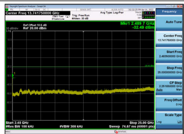
,Plot 4,2483.5MHz~25000MHz-802.11n(HT40),2452MHz,Ant0
