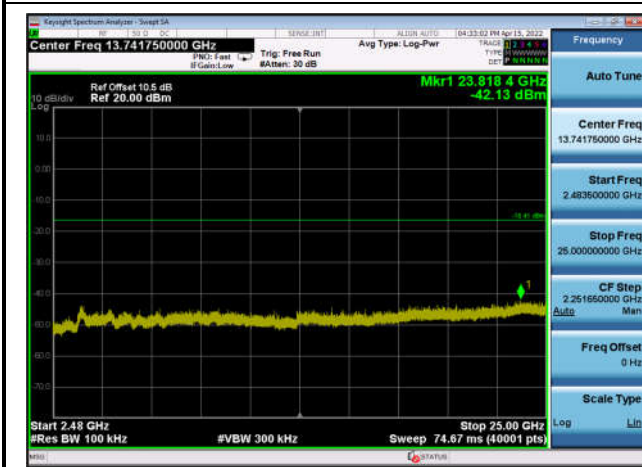
,Plot 4,2483.5MHz~25000MHz-802.11n(HT20),2437MHz,Ant1
