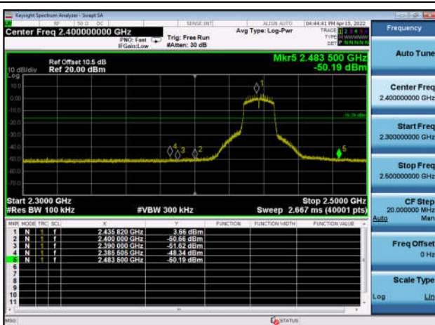
,Plot 2,Band Edge-802.11ax(HE20) ,2437MHz,Ant0
