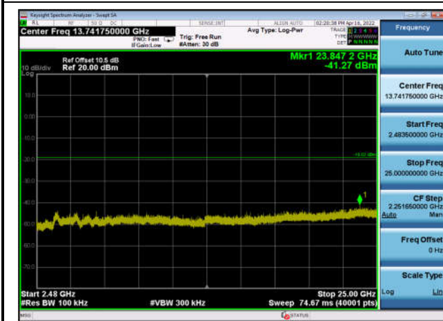
,Plot 4,2483.5MHz~25000MHz-802.11n(HT40),2437MHz,Ant0
