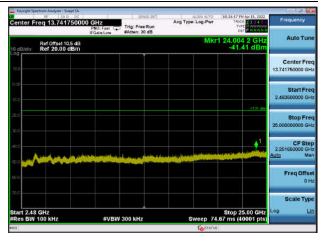
,Plot 4,2483.5MHz~25000MHz-802.11n(HT20),2462MHz,Ant1
