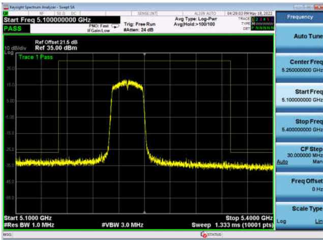
U-NII-1 ,802.11ax-HE40, 5190MHz, Ant4
