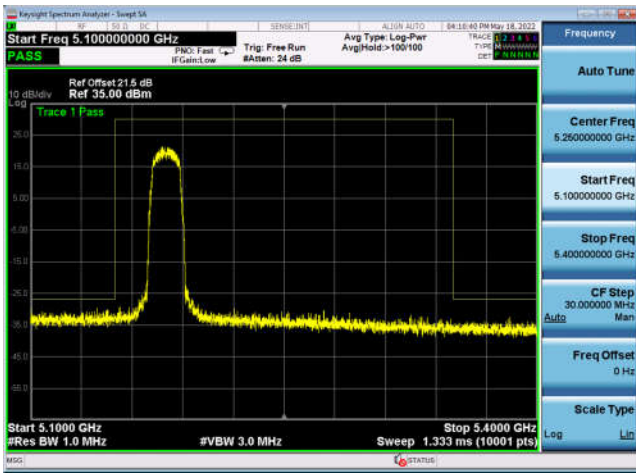
U-NII-1 ,802.11a, 5220MHz, Ant5
