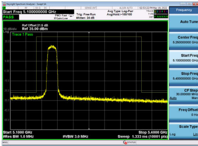
U-NII-1 ,802.11a, 5220MHz, Ant0
