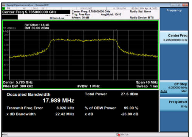
U-NII-3 99% OBW & 26 EBW-802.11n(20MHz) ,5785MHz,Ant2
