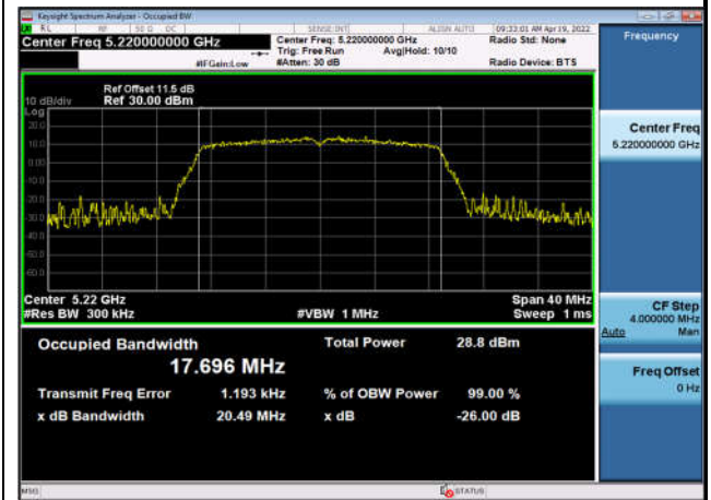
U-NII-1 99% OBW & 26 EBW-802.11ac(20MHz) ,5220MHz,Ant4
