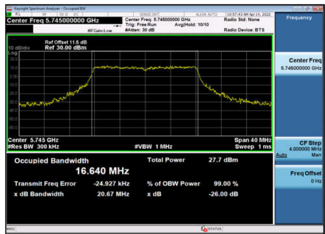
U-NII-3 99% OBW & 26 EBW-802.11a(20MHz) ,5745MHz,Ant0
