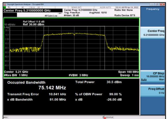
U-NII-1 99% OBW & 26 EBW-802.11ax(80MHz) ,5210MHz,Ant5
