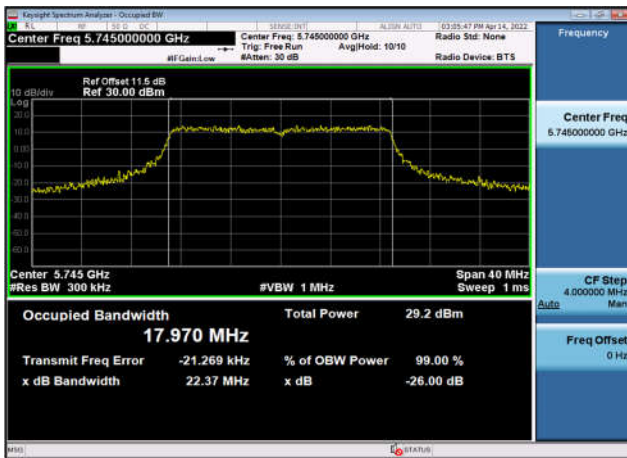
U-NII-3 99% OBW & 26 EBW-802.11ac(20MHz) ,5745MHz,Ant1
