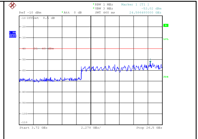
15MHz - Low CH 3.72GHz~26.5GHz
