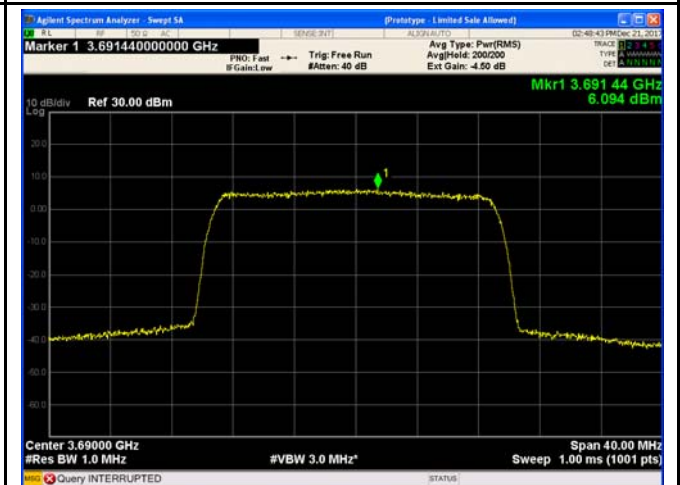
20MHz - High CH 16QAM
