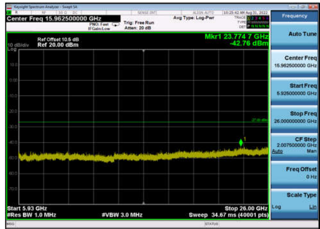
U-NII-3 ,Plot 3,5925MHz~26000MHz-802. 11ax(20MHz),5785MHz,Ant1
