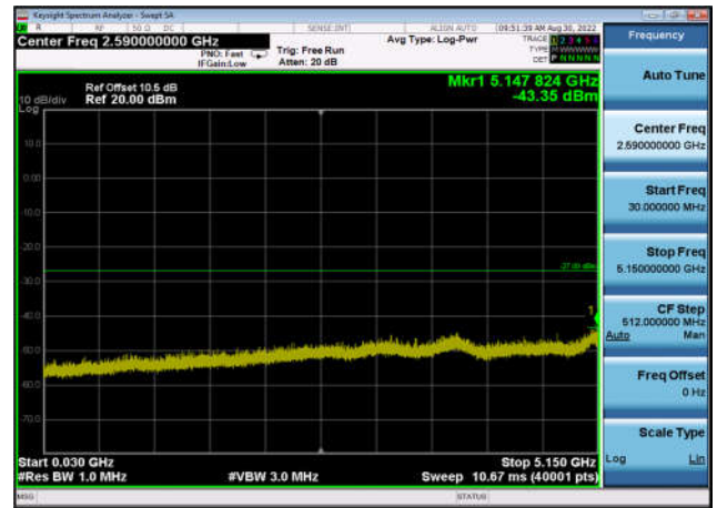
U-NII-1 ,Plot 2,30MHz~5150MHz-802.11a x(40MHz),5230MHz,Ant1
