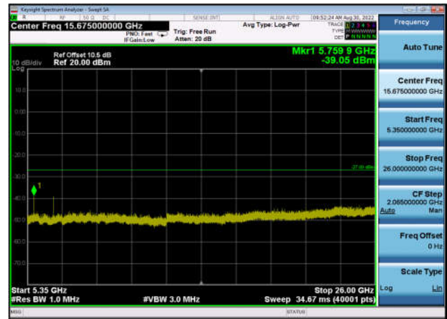
U-NII-1 ,Plot 3,5350MHz~26000MHz-802. 11ax(40MHz),5230MHz,Ant1
