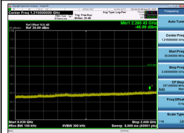
,Plot 3,30MHz~2400MHz-802.11ax(HE40) ,2452MHz,Ant0
