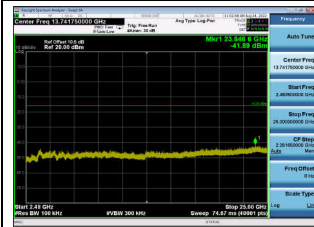
,Plot 4,2483.5MHz~25000MHz-802.11ax(H T20),2437MHz,Ant0
