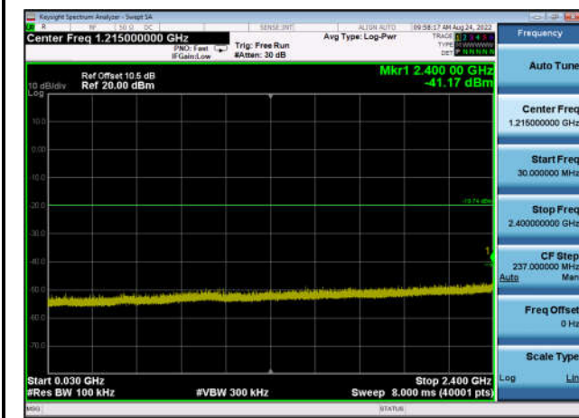
,Plot 3,30MHz~2400MHz-802.11n(HT40) ,2437MHz,Ant0
