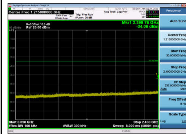
,Plot 3,30MHz~2400MHz-802.11n(HT20) ,2437MHz,Ant0
