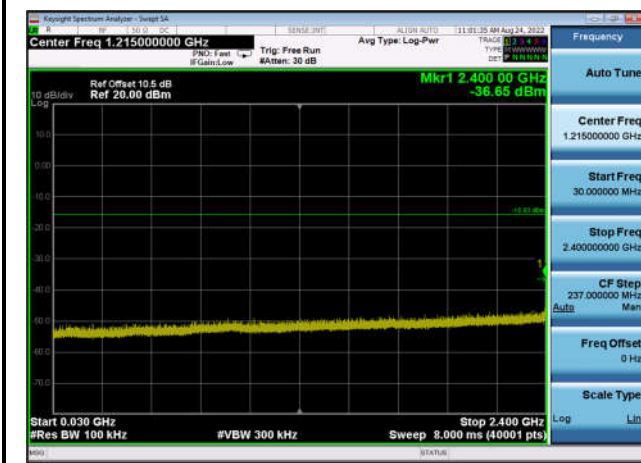
,Plot 3,30MHz~2400MHz-802.11ax(HE20) ,2437MHz,Ant0
