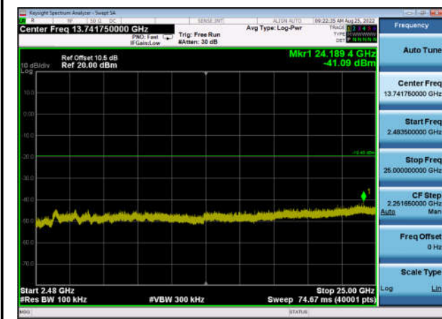
,Plot 4,2483.5MHz~25000MHz-802.11ax(H T40),2437MHz,Ant0
