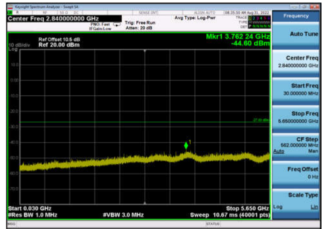
U-NII-3 ,Plot 2,30MHz~5650MHz-802.11n (20MHz),5785MHz,Ant1
