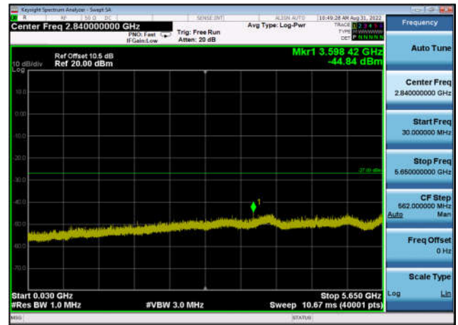
U-NII-3 ,Plot 2,30MHz~5650MHz-802.11a x(40MHz),5795MHz,Ant1
