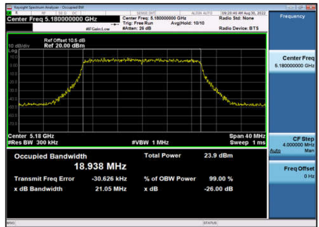
U-NII-1 99% OBW & 26dB EBW-802.11ax(20MHz) ,5180MHz,Ant1
