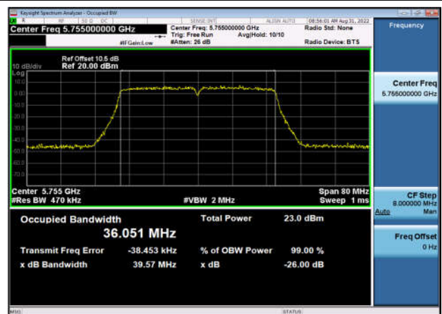
U-NII-3 99% OBW & 26dB EBW-802.11n(40MHz) ,5755MHz,Ant1
