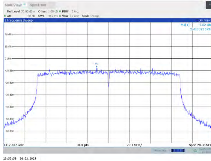
11ax20MIMO_Ant1_2437
