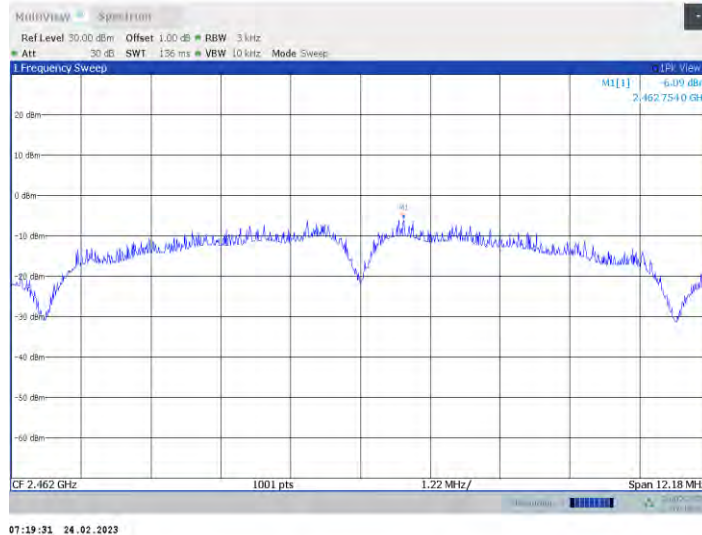
11b-CDD_Ant1_2462
