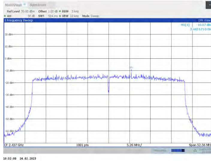
11ax40MIMO_Ant1_2437
