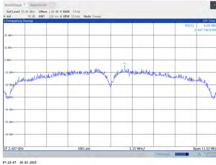
11b-CDD_Ant1_2437
