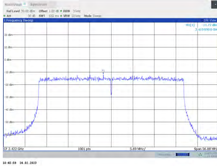
11ax40MIMO_Ant1_2422
