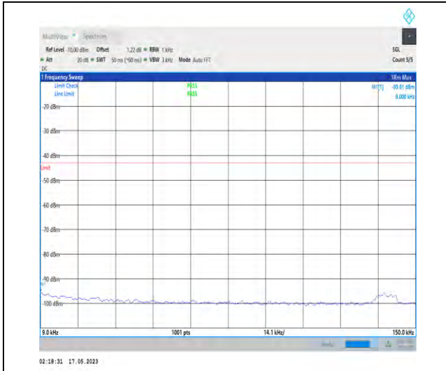
1-N66-PC3-15-30-H-1-DFT-PI2BPSK-Inner_1RB_L eft-1@1-0.009-0.15-Ant1-0.01--95.61--43-PASS
