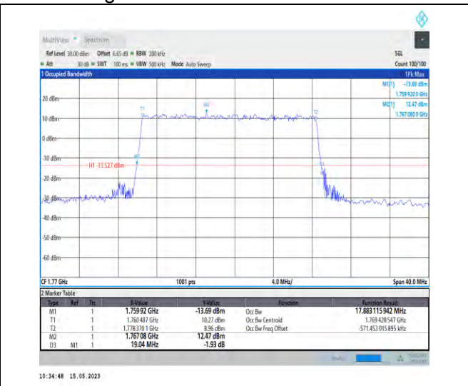
1-DC_5A_n66A-PC3-15-5+20-M+H-3-N/A-N/A-N/A-DFT-16QAM-Outer_Full-100@0-Ant1-17.883-19.040 -≤20-PASS
