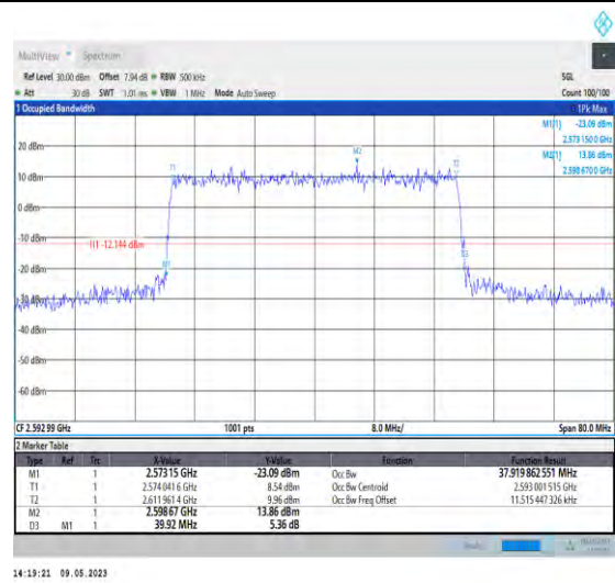
1-N41-PC3-30-40-M-7-CP-16QAM-Outer_Full-106@ 0-Ant1-37.92-39.920-≤40-PASS
