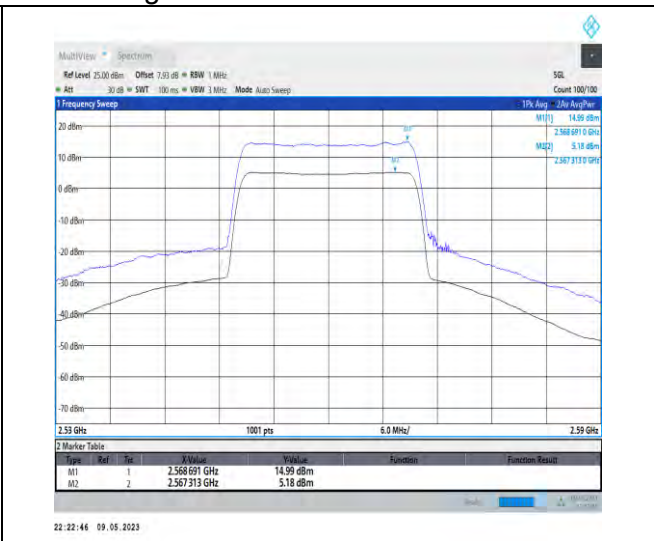
1-N7-PC3-15-20-H-2-CP-256QAM-Outer_Full-106@ 0-Ant1-9.81-100%-0.00-9.81-PASS-≤13
