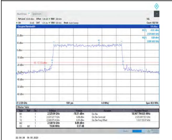
1-N7-PC3-15-20-M-9-CP-256QAM-Outer_Full-106@0 0-Ant1-18.948-19.840-≤20-PASS
