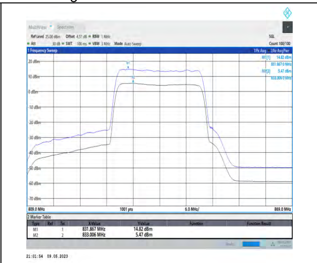
1-N5-PC3-15-20-H-2-CP-256QAM-Outer_Full-106@ 0-Ant1-9.35-100%-0.00-9.35-PASS-≤13
