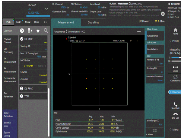
38-38-20MHz-20MHz-16QAM-16QAM -37901-38099-100RB#0-100RB#0
