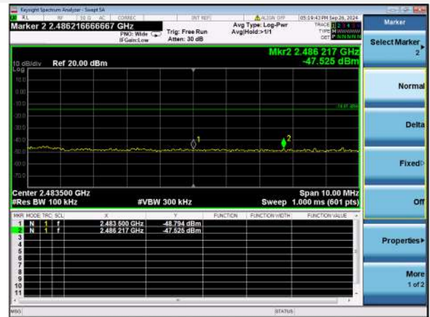
802.11b CH11, BAND EDGE
