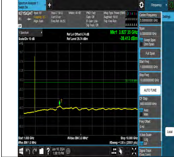
Band2 10MHz QPSK 18650 50RB#0 1000~1000 1000~1000
