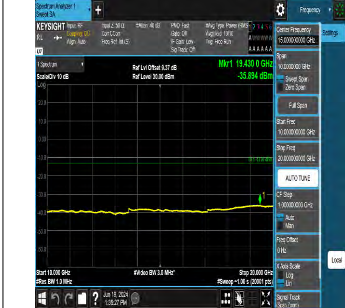
Band2 20MHz QPSK 19100 100RB#0 10000~20000 10000~20000
