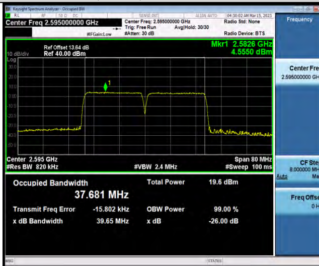
38-38-20MHz-20MHz-QPSK-QPSK-37952-38150-100RB#0-100RB#0
