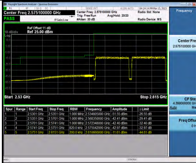
38-38-20MHz-20MHz-16QAM-16QAM-37901-38099-1RB#0-0RB#0
