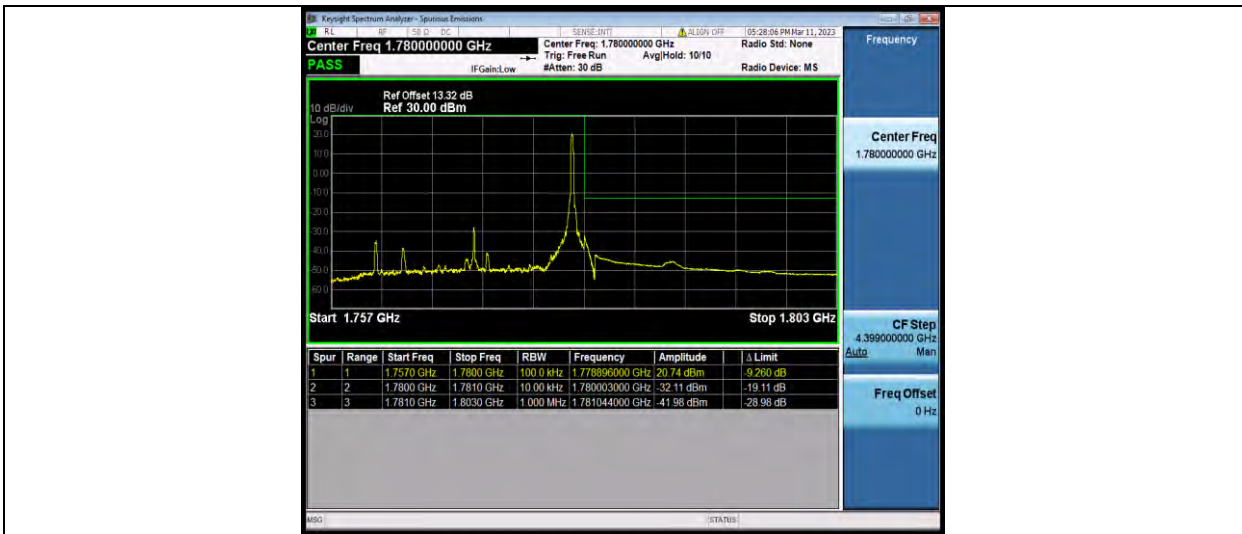
Band66-20MHz-QPSK-132572-100RB#0
