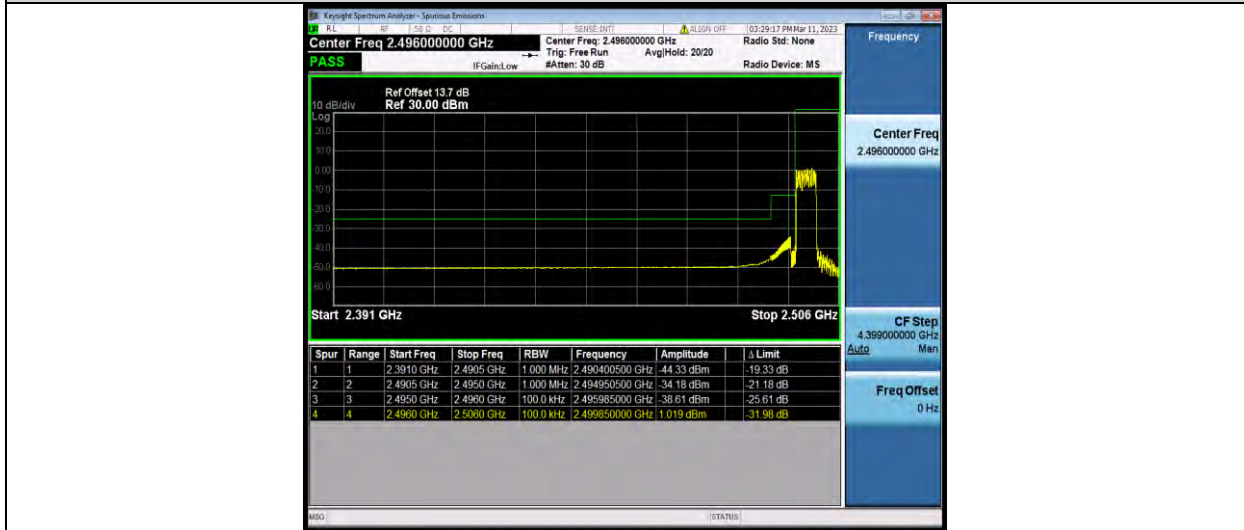
Band41-5MHz-64QAM-41565-1RB#24
