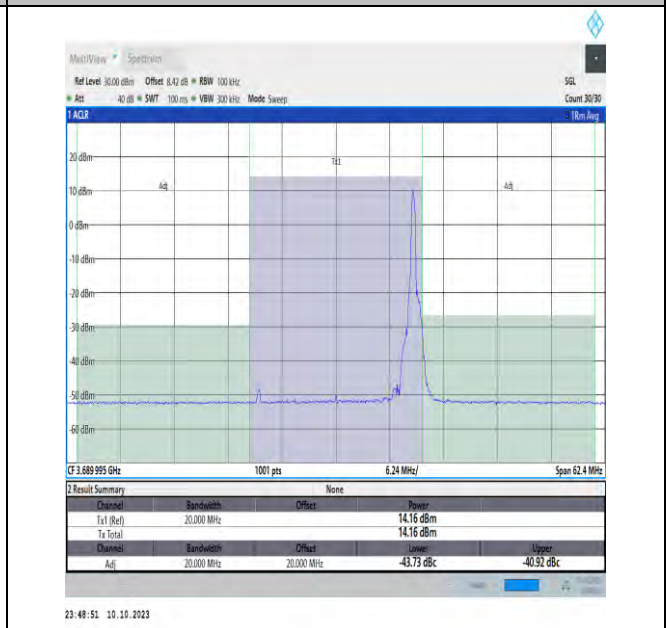
NTVN_N48_PC3_30_20_H_TID18_#1_-20_20
