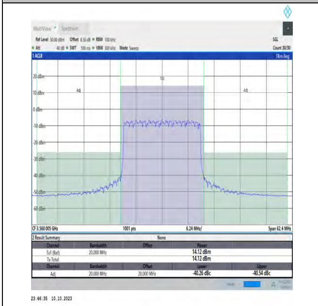
NTVN_N48_PC3_30_20_L_TID16_#1_-20_20
