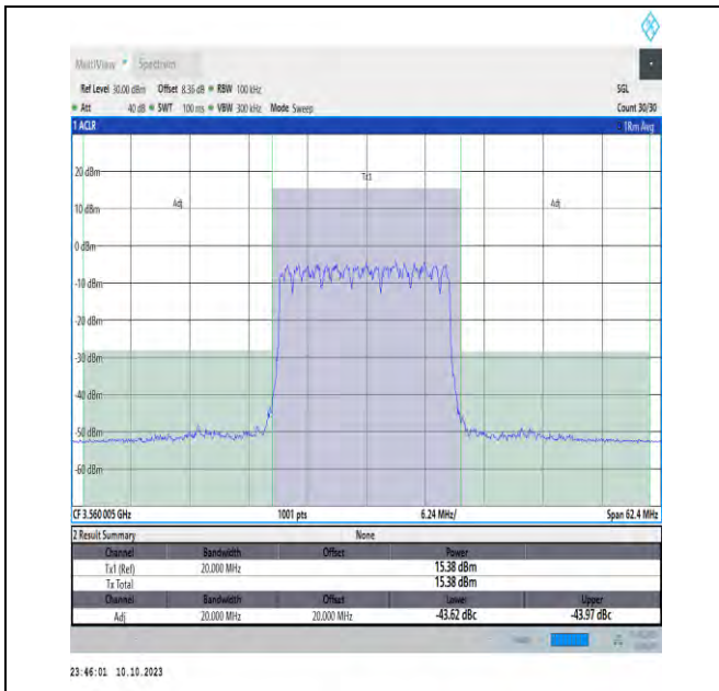
NTVN_N48_PC3_30_20_L_TID1_#1_-20_20
