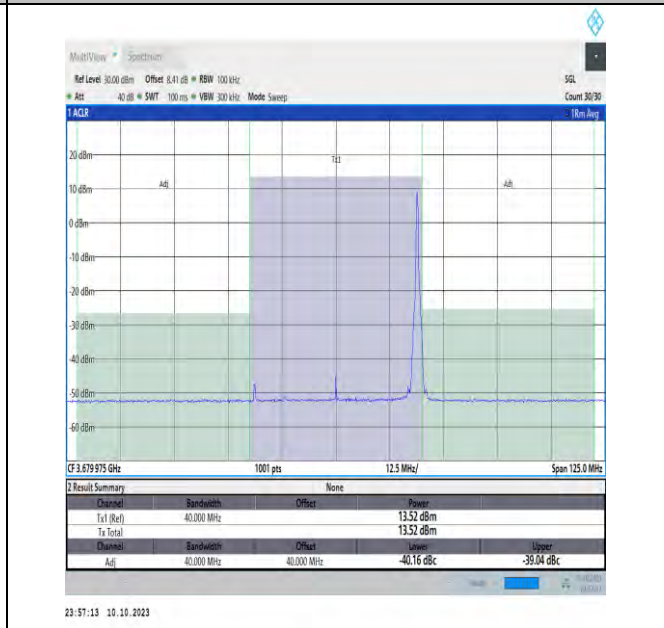
NTVN_N48_PC3_30_40_H_TID18_#1_-40_40
