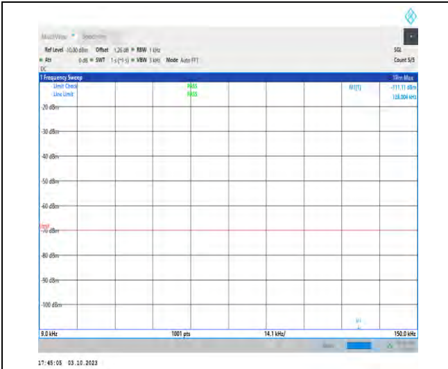
1-N48-PC3-30-40-H-1-DFT-PI2BPSK-Inner_1RB_L eft-1@1-0.009-0.15-Ant7-0.06--83.74--70-PASS
