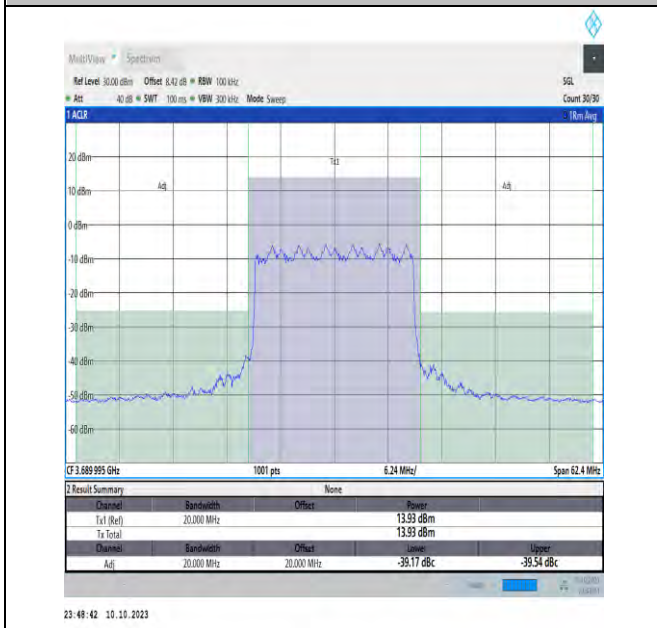
NTVN_N48_PC3_30_20_H_TID16_#1_-20_20
