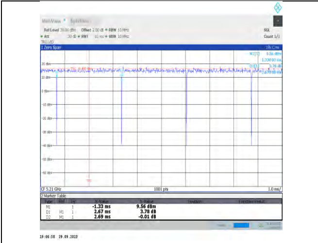
NTNV-11ax80MIMO-Ant6-5210
