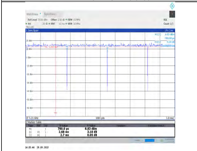
NTNV-11be80MIMO-Ant6-5210
