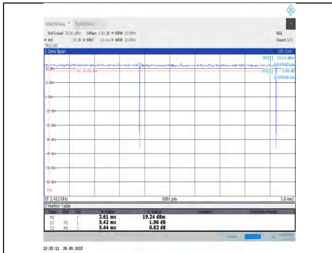
NTVN-11be20MIMO-Ant16-2412
