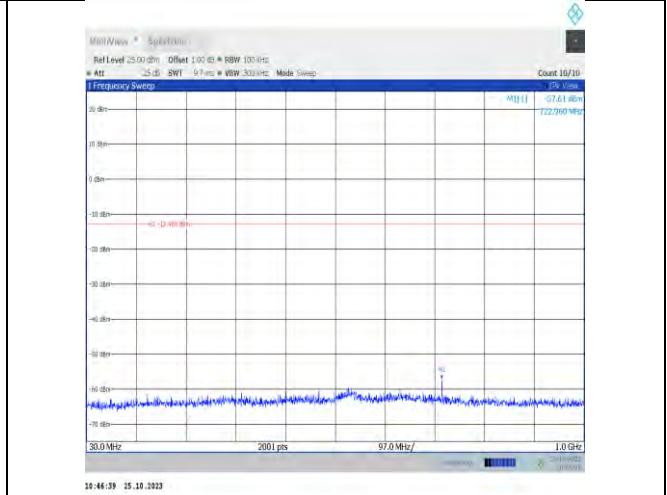
11n20MIMO-Ant16-2437-30~1000-PASS
