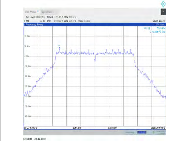
11g-CDD-Ant16-2462-0~Reference-PASS
