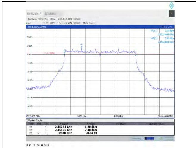
11be20MIMO-Ant16-2462-PASS
