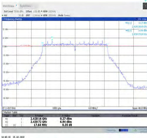
11n20MIMO-Ant16-2437-PASS
