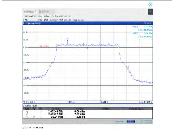
11be20MIMO-Ant16-2412-PASS
