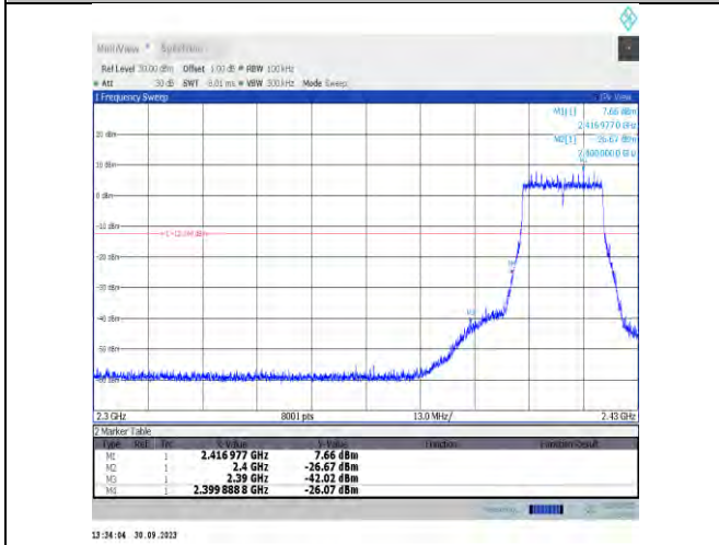
11be20MIMO-Ant16-2412-PASS
