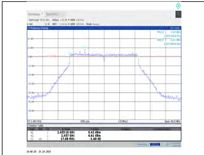
11n20MIMO-Ant16-2462-PASS
