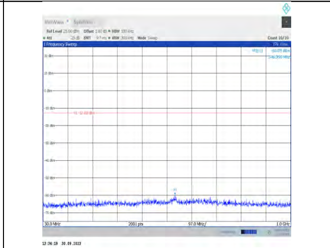
11be20MIMO-Ant16-2412-30~1000-PASS
