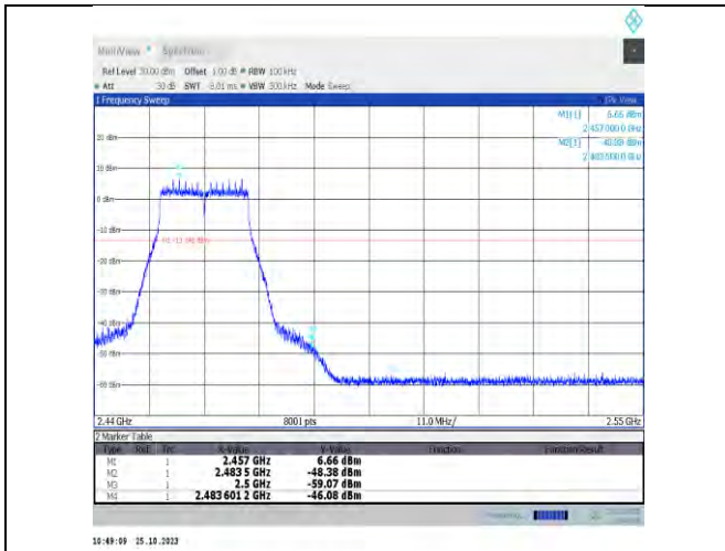
11n20MIMO-Ant16-2462-PASS
