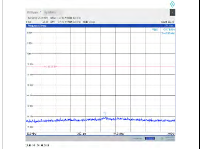
11be20MIMO-Ant16-2437-30~1000-PASS
