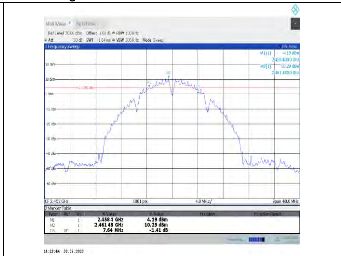
11b-CDD-Ant7-2462-PASS
