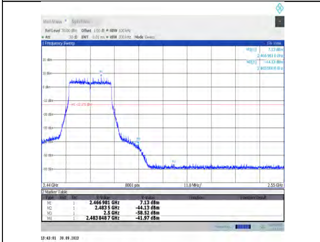
11be20MIMO-Ant16-2462-PASS
