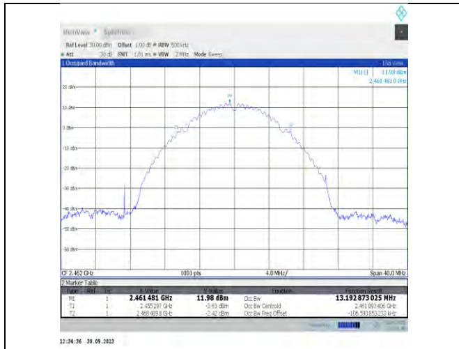
11b-CDD-Ant16-2462
