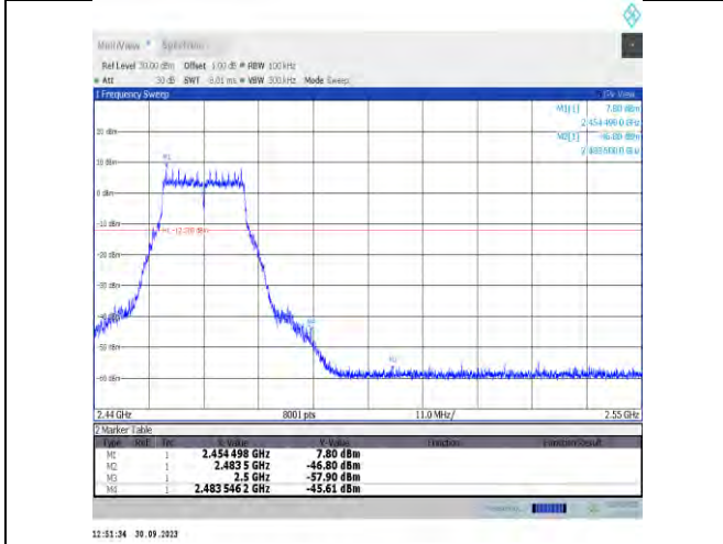
11g-CDD-Ant16-2462-PASS
