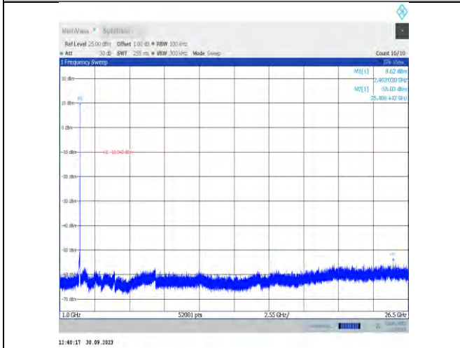
11b-CDD-Ant16-2462-1000~26500-PASS
