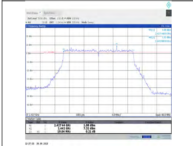
11be20MIMO-Ant16-2437-PASS
