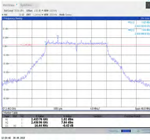
11g-CDD-Ant16-2462-PASS
