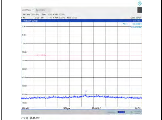
11n20MIMO-Ant16-2412-30~1000-PASS
