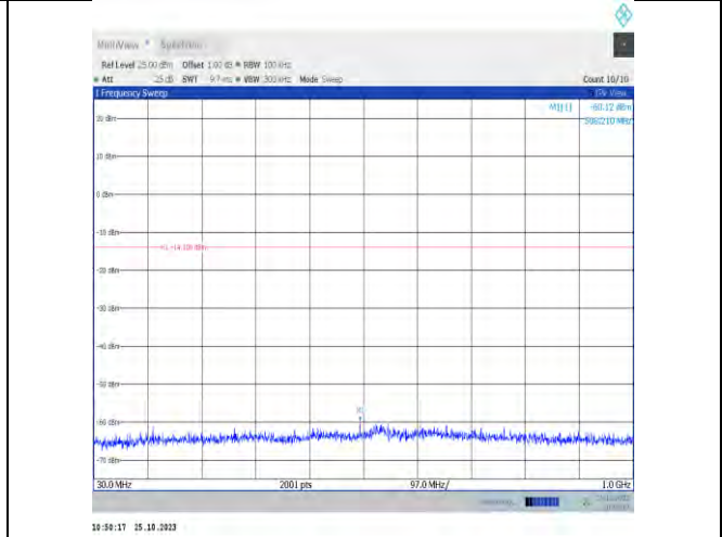
11n20MIMO-Ant16-2462-30~1000-PASS
