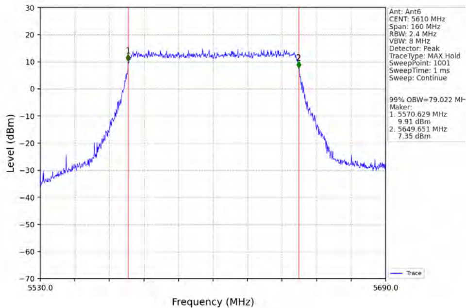
802.11ax(HEW80) HCH 5610MHz RU996 Left Ant6 NTN
