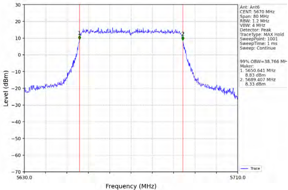
802.11be(EHT40)_HCH_5670MHz_RU484_Left_Ant6_NTNV
