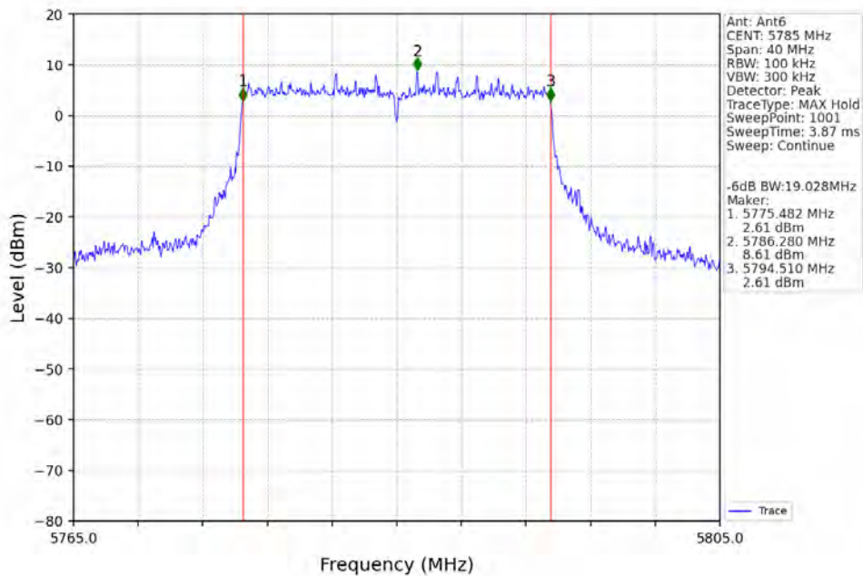
802.11be(EHT20)_MCH_5785MHz_RU242_Left_Ant6_NTNV
