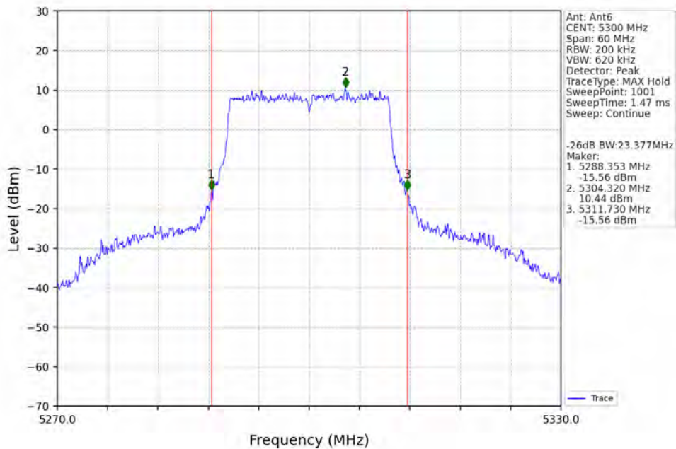
802.11be(EHT20)_MCH_5300MHz_RU242_Left_Ant6_NTNV
