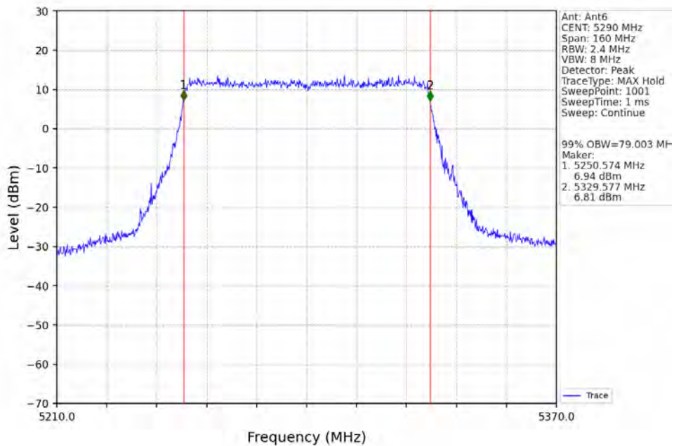
802.11ax(HEW80)_MCH_5290MHz_RU996_Left_Ant6_NTNV
