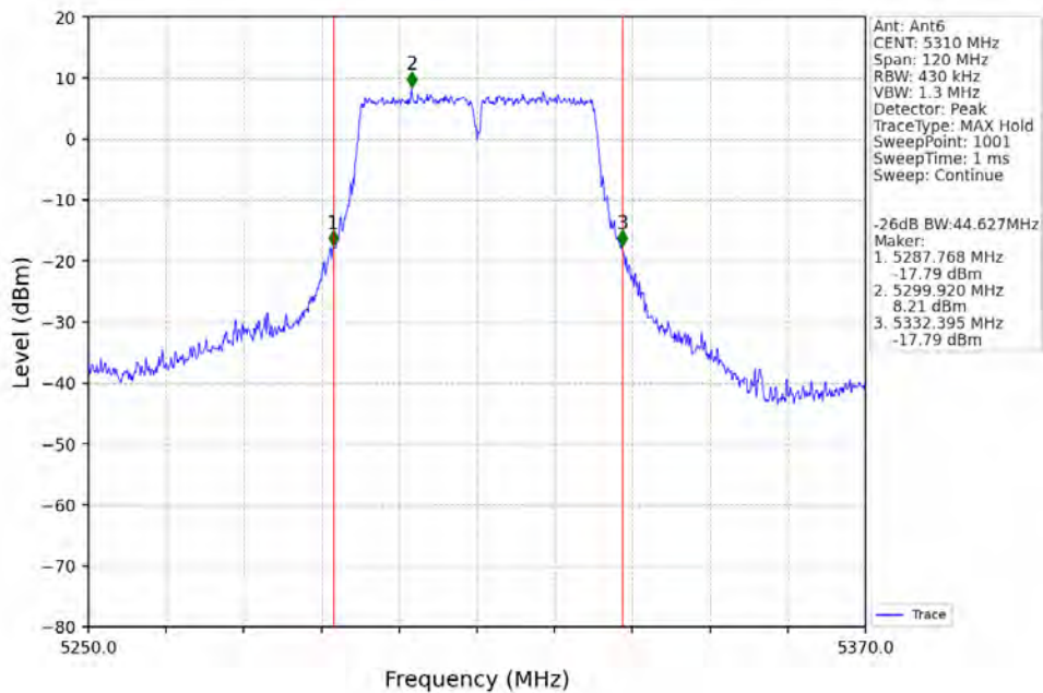
802.11ac(VHT40) HCH 5310MHz_Ant6_NTNV
