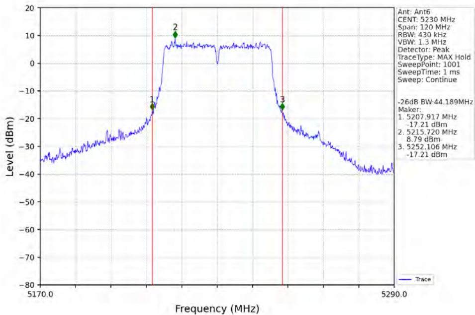
802.11n(HT40)_HCH_5230MHz_Ant6_NTNV
