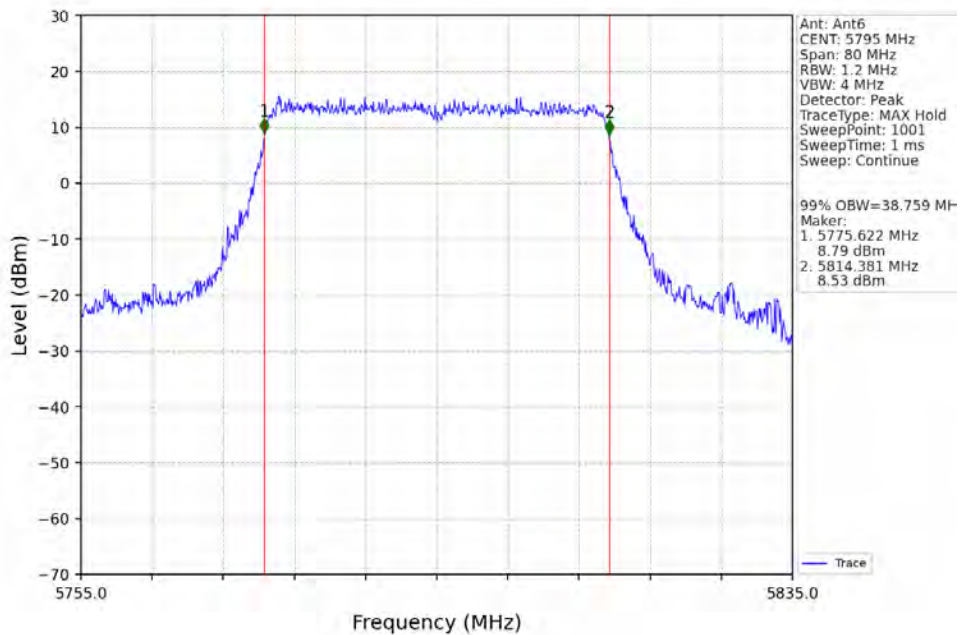
802.11be(EHT40)_HCH_5795MHz_RU484_Left_Ant6_NTNV
