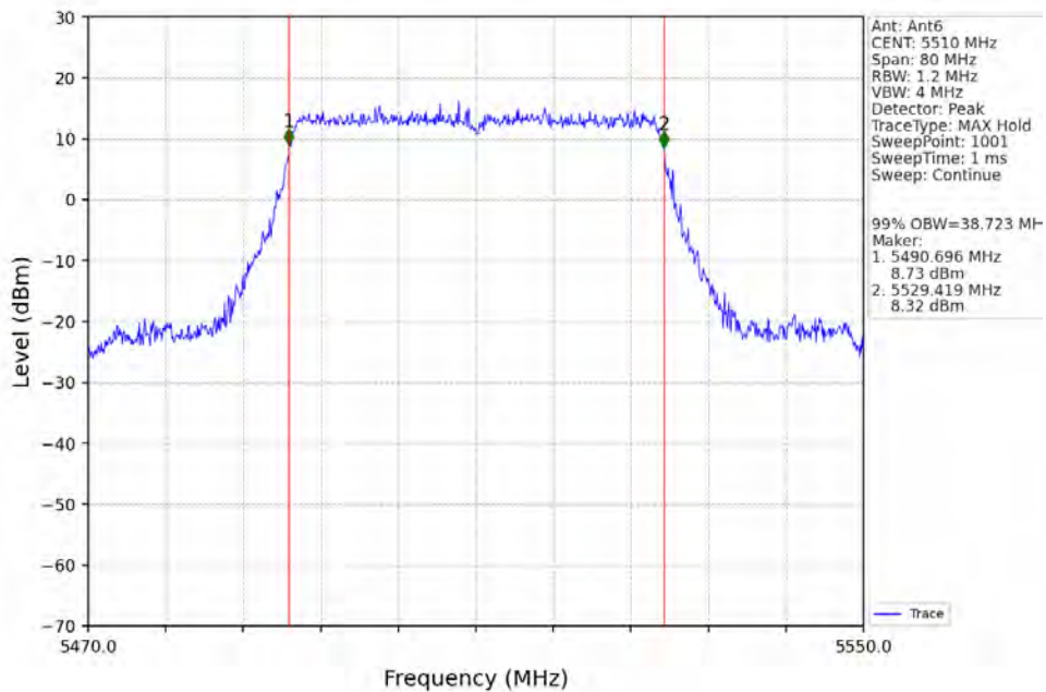
802.11be(EHT40)_LCH_5510MHz_RU484_Left_Ant6_NTNV
