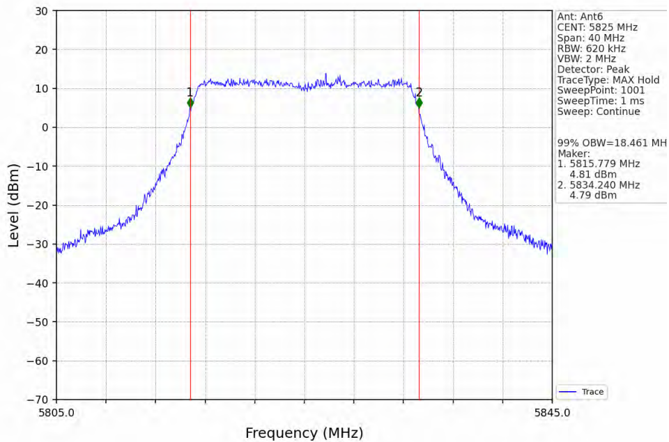
802.11n(HT20)_HCH_5825MHz_Ant6_NTNV
