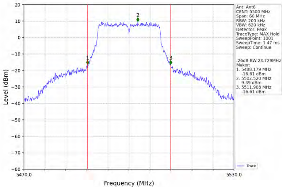
802.11ac(VHT20)_LCH_5500MHz_Ant6_NTNV
