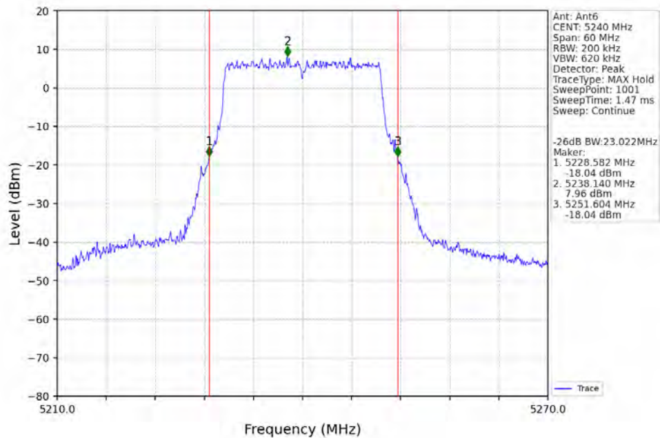
802.11be(EHT20)_HCH_5240MHz_RU242_Left_Ant6_NTNV
