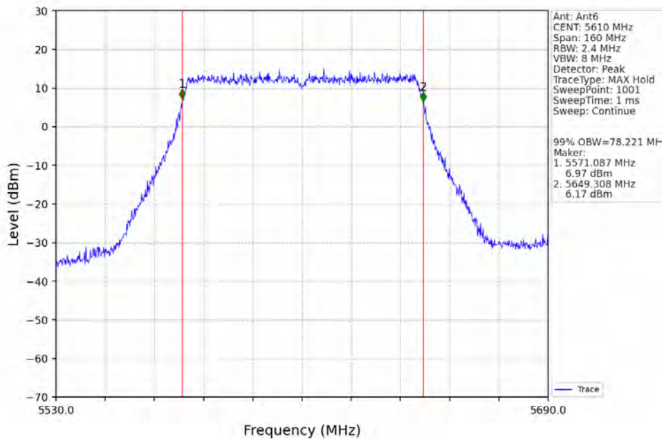
802.11ac(VHT80) HCH 5610MHz_Ant6_NTNV
