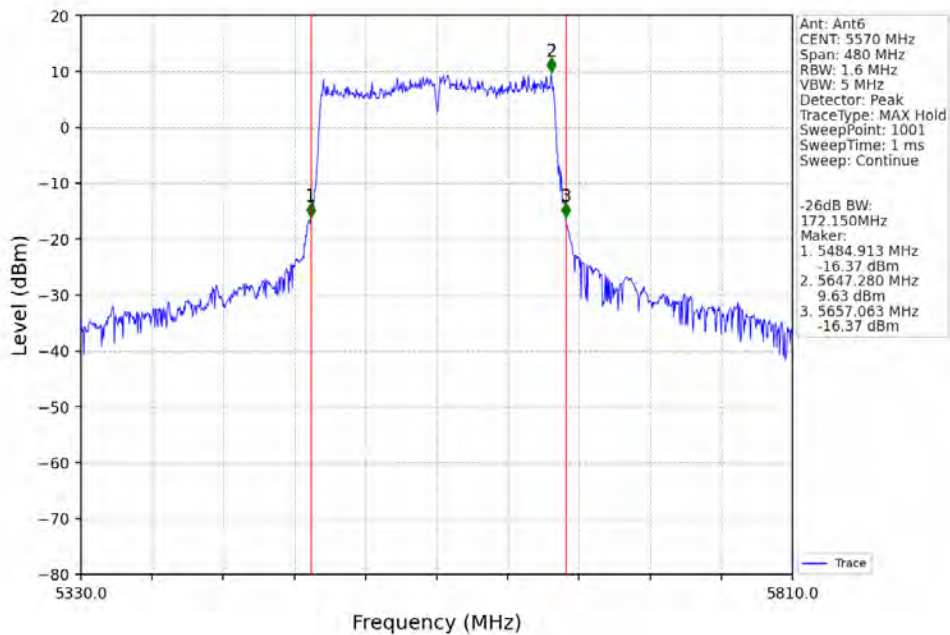
802.11ax(HEW160)_MCH_5570MHz_2xRU996_Left_Ant6_NTNV
