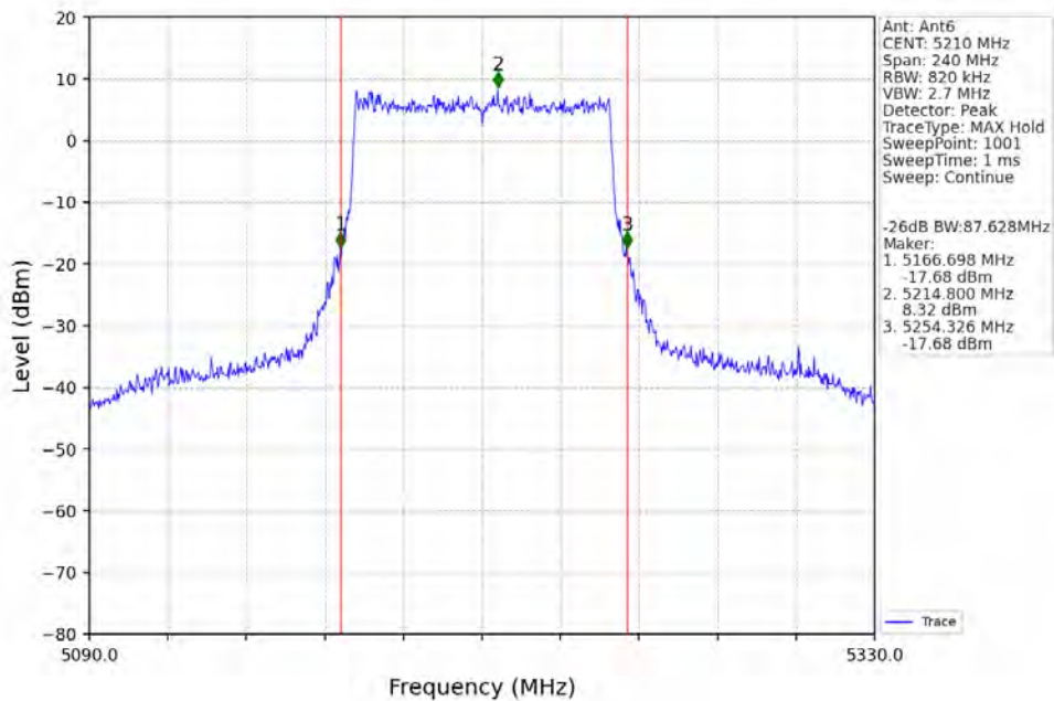
802.11ax(HEW80)_MCH_5210MHz_RU996_Left_Ant6_NTNV
