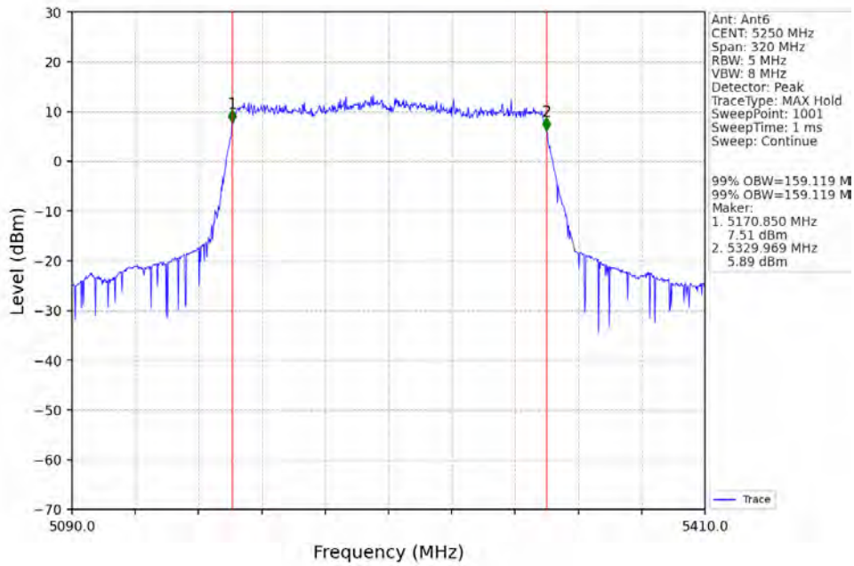
802.11be(EHT160)_MCH_5250MHz_2xRU996_Left_Ant6_NTNV
