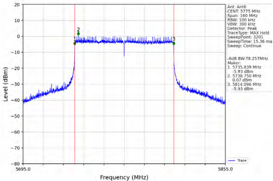
802.11be(EHT80)_MCH_5775MHz_RU996_Left_Ant6_NTNV
