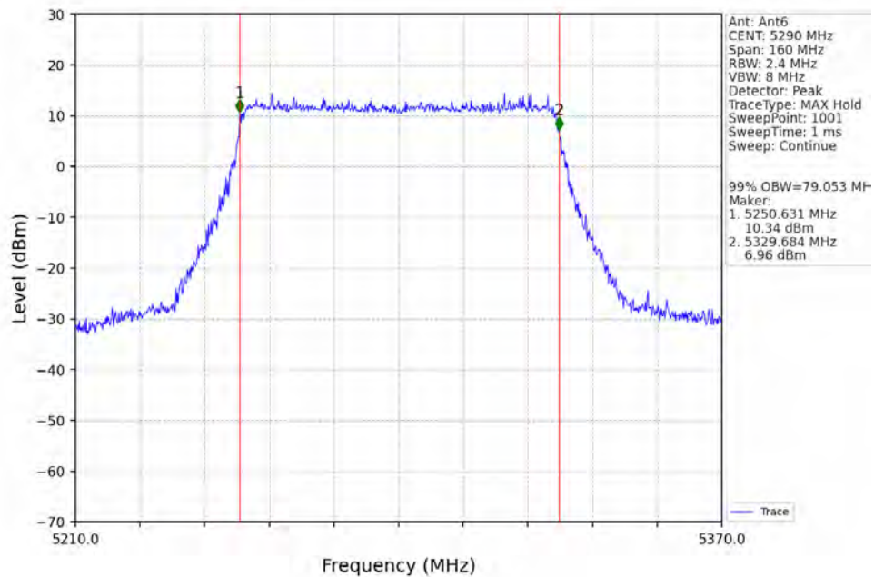
802.11be(EHT80)_MCH_5290MHz_RU996_Left_Ant6_NTNV
