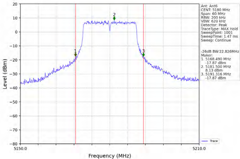
802.11n(HT20)_LCH_5180MHz_Ant6_NTNV
