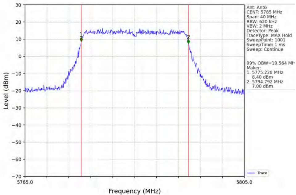
802.11be(EHT20)_MCH_5785MHz_RU242_Left_Ant6_NTNV
