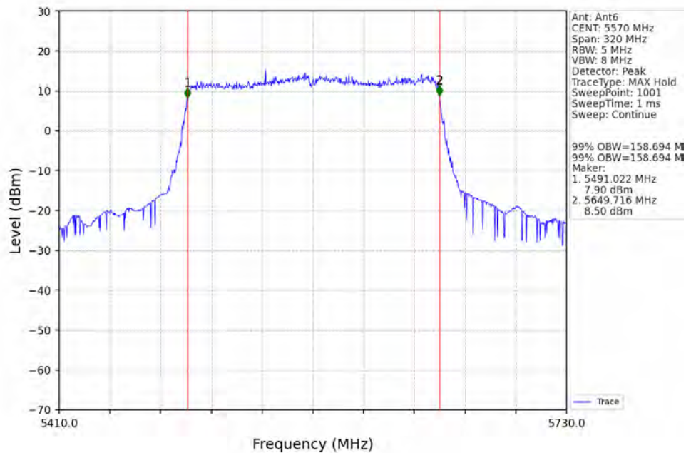
802.11ax(HEW160)_MCH_5570MHz_2xRU996_Left_Ant6_NTNV
