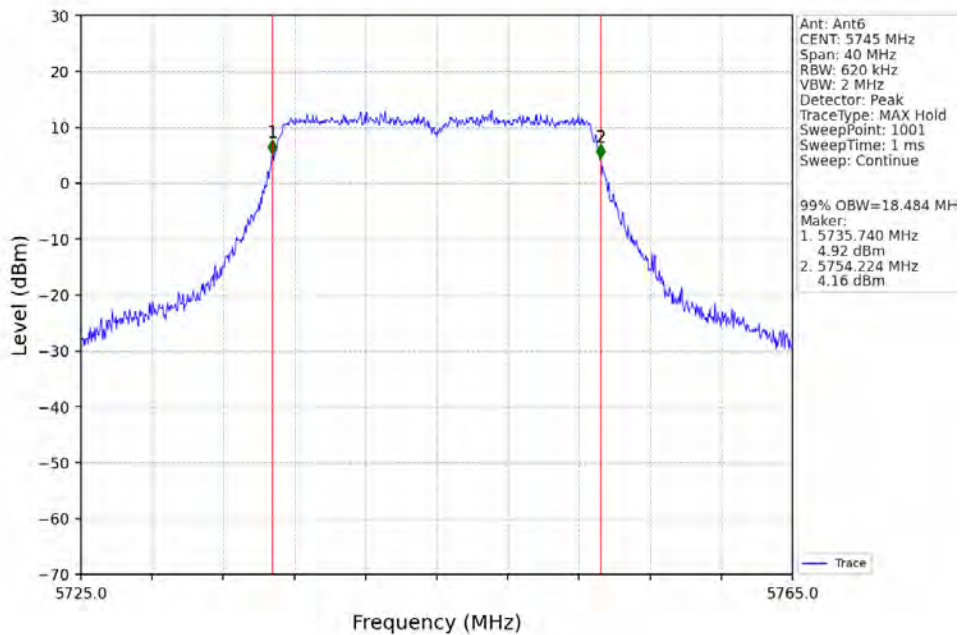
802.11n(HT20)_LCH_5745MHz_Ant6_NTNV
