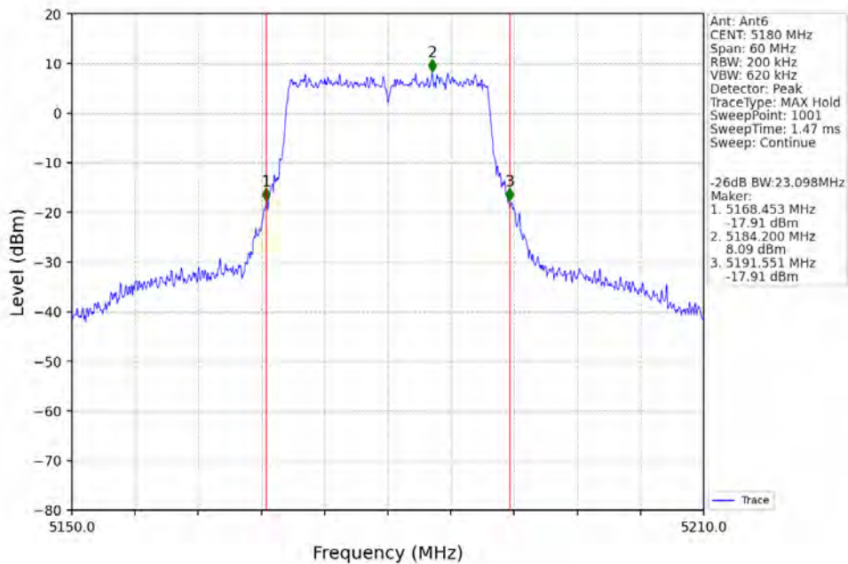
802.11be(EHT20)_LCH_5180MHz_RU242_Left_Ant6_NTNV
