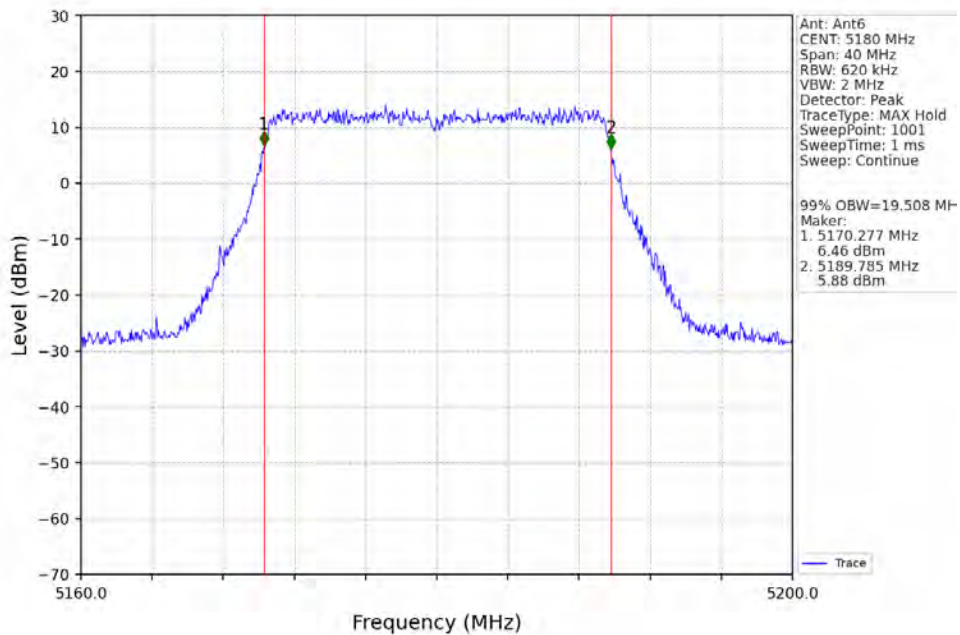
802.11be(EHT20)_LCH_5180MHz_RU242_Left_Ant6_NTNV
