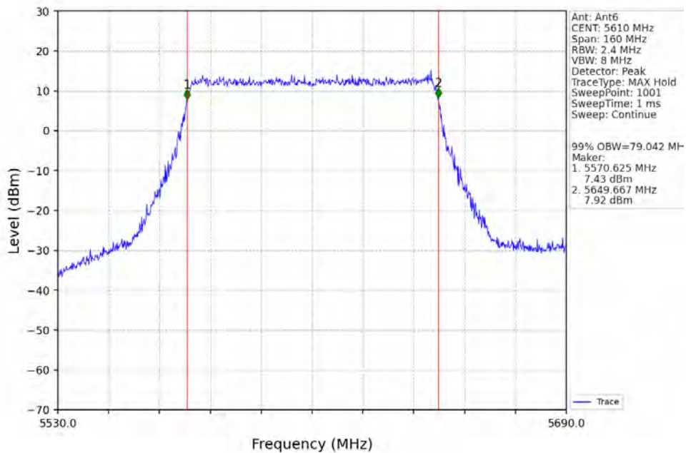
802.11be(EHT80)_HCH_5610MHz_RU996_Left_Ant6_NTNV
