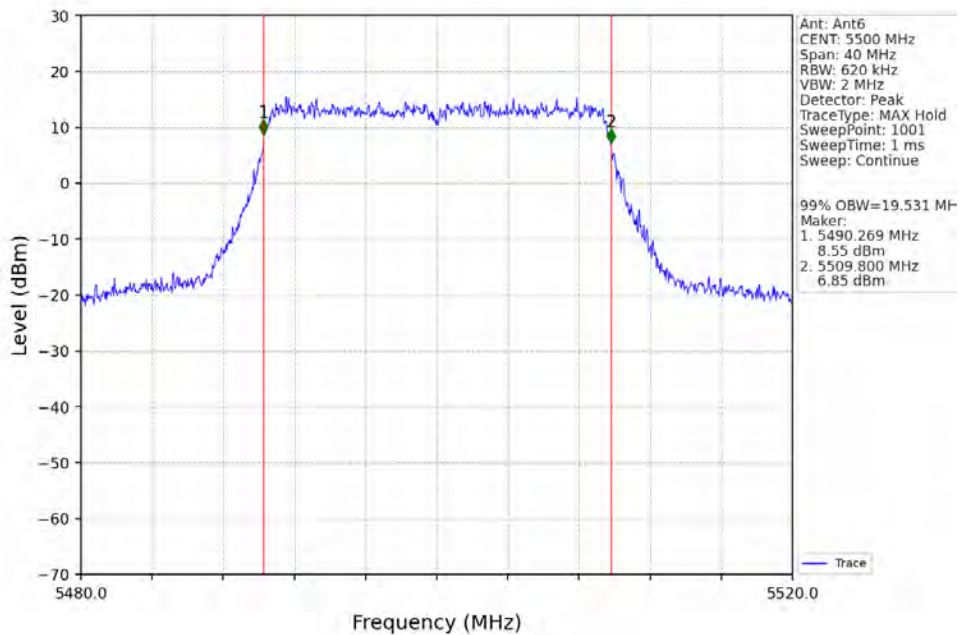
802.11ax(HEW20) LCH_5500MHz_RU242_Left_Ant6_NTNV
