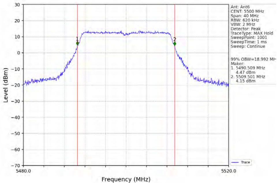
802.11ac(VHT20)_LCH_5500MHz_Ant6_NTNV
