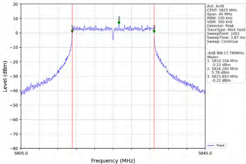
802.11n(HT20)_HCH_5825MHz_Ant6_NTNV
