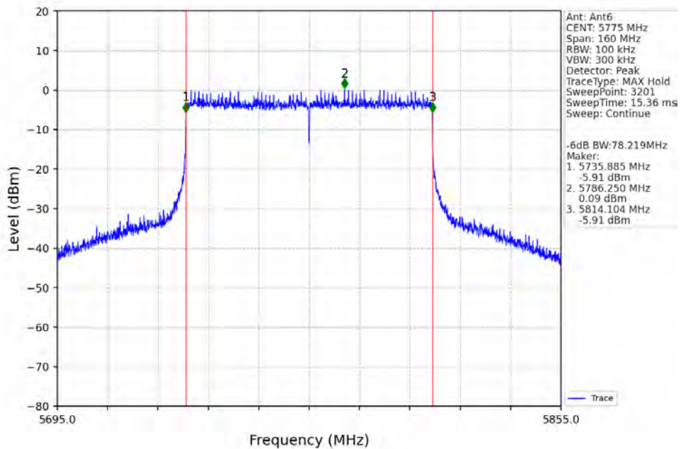
802.11ax(HEW80)_MCH_5775MHz_RU996_Left_Ant6_NTNV
