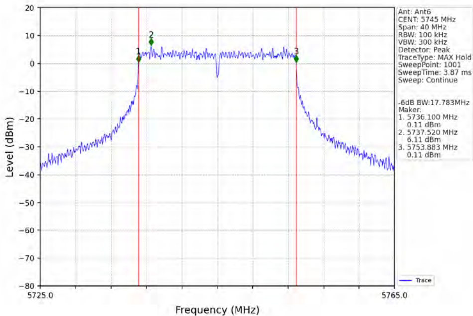
802.11n(HT20)_LCH_5745MHz_Ant6_NTNV
