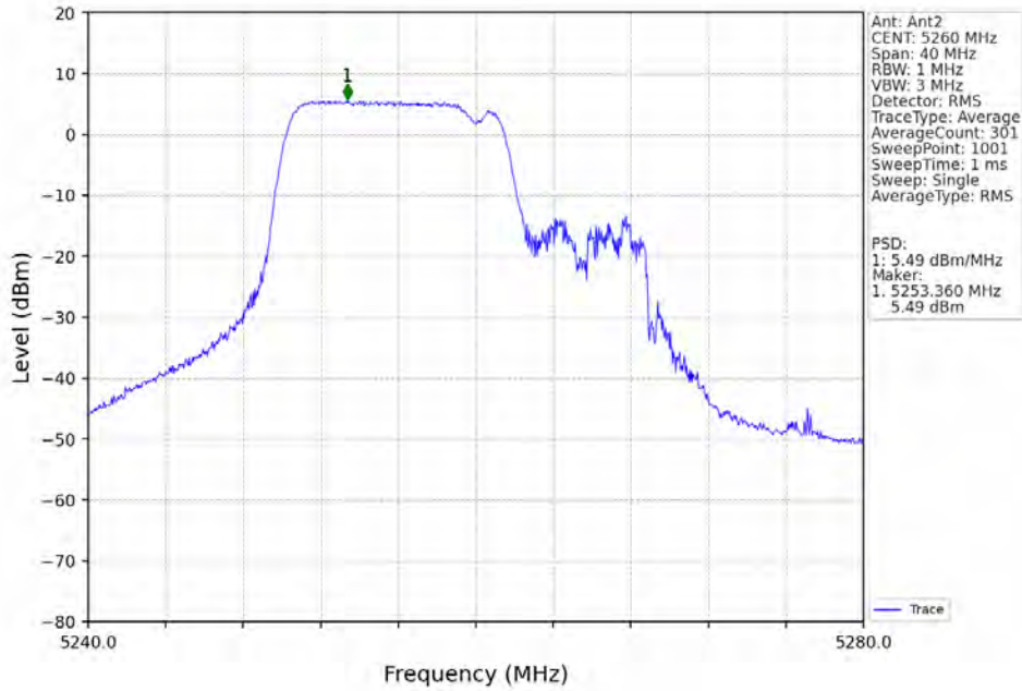
802.11be(EHT20)_LCH_5260MHz_RU106_Left_MIMO_NTNV
