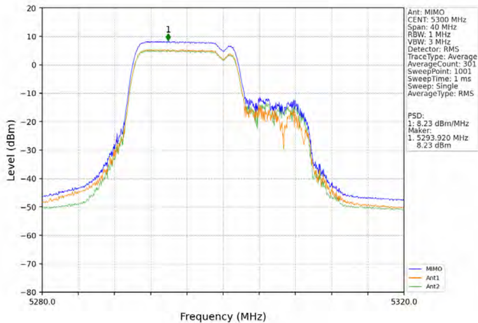
802.11be(EHT20)_MCH_5300MHz_RU106_Left_MIMO_NTNV
