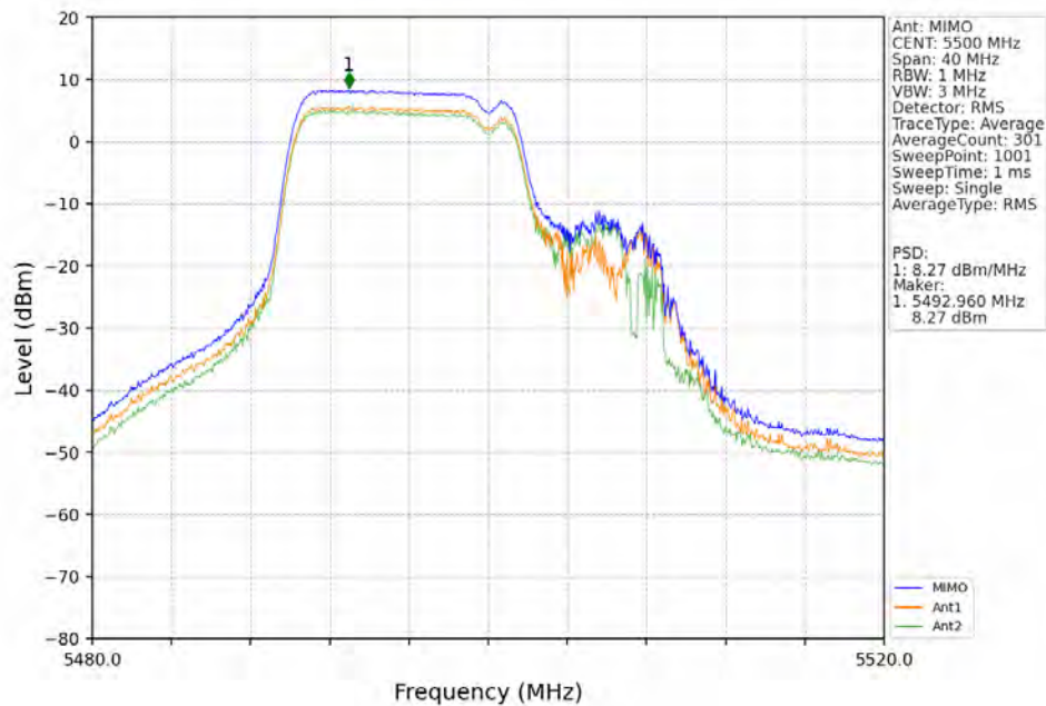
802.11be(EHT20)_LCH_5500MHz_RU106_Left_MIMO_NTNV
