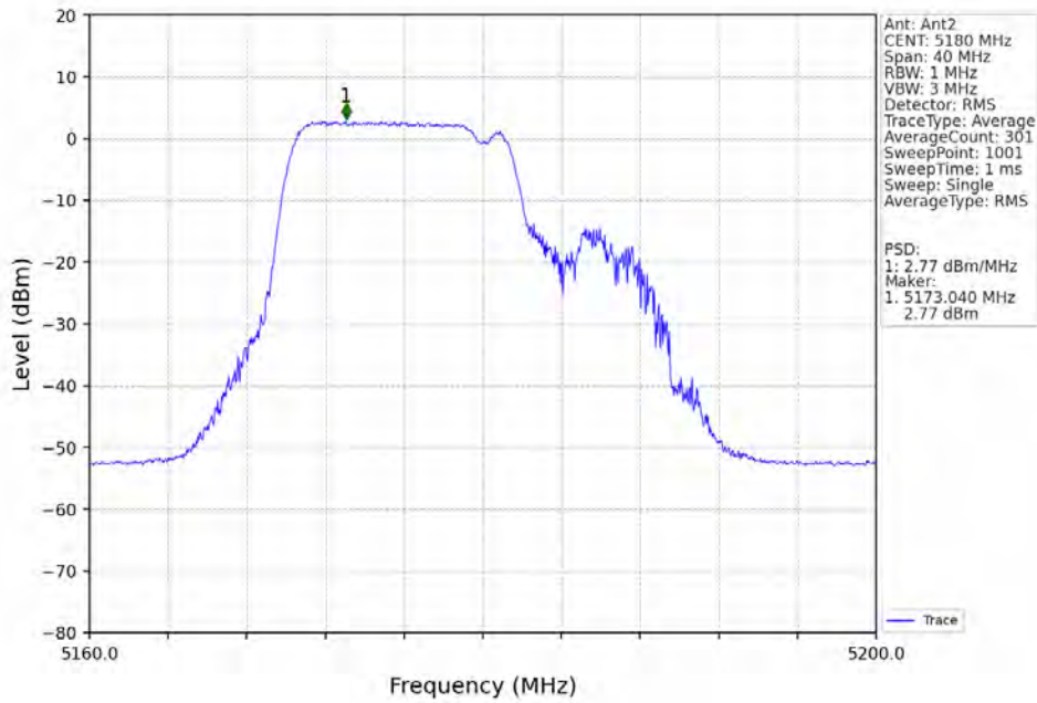
802.11be(EHT20)_LCH_5180MHz_RU106_Left_MIMO_NTNV
