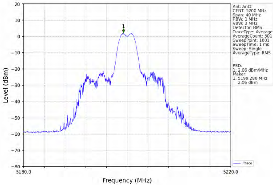
802.11be(EHT20)_MCH_5200MHz_RU26_Mid_MIMO_NTNV
