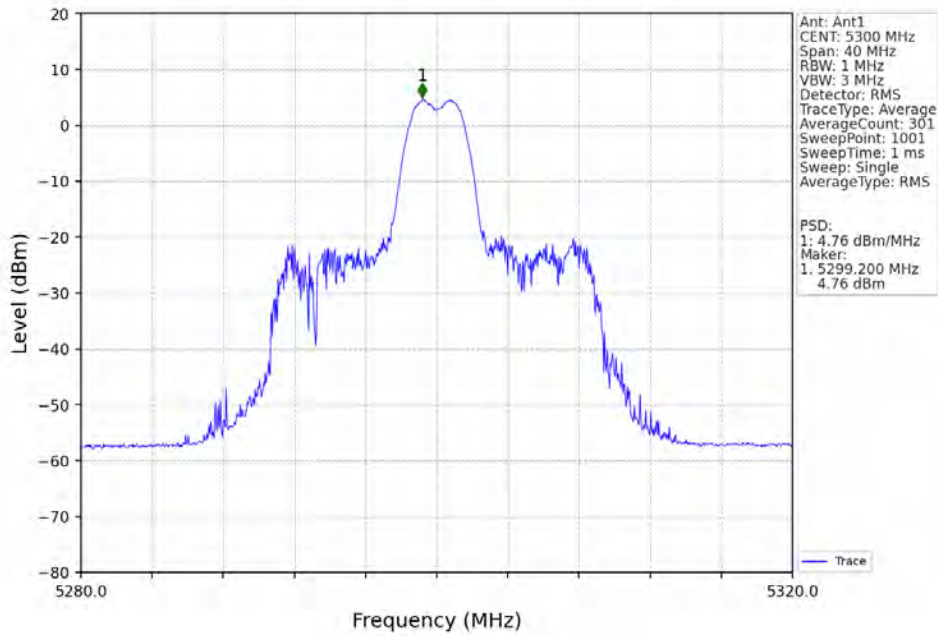
802.11be(EHT20)_MCH_5300MHz_RU26_Mid_Ant17_NTNV
