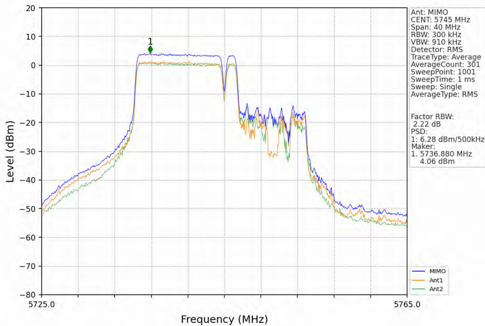
802.11be(EHT20)_LCH_5745MHz_RU106_Left_MIMO_NTNV
