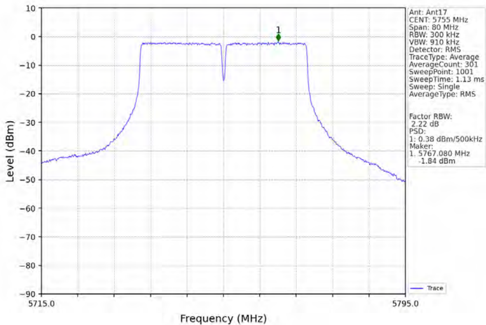
802.11n(HT40)_LCH_5755MHz_Ant17_NTNV
