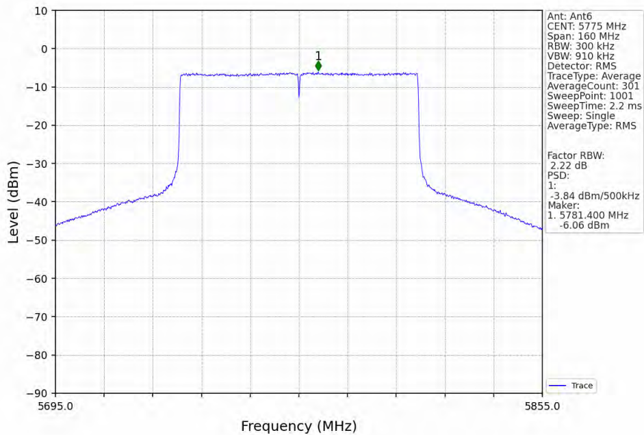
802.11be(EHT80)_MCH_5775MHz_RU996_Left_Ant6_NTNV
