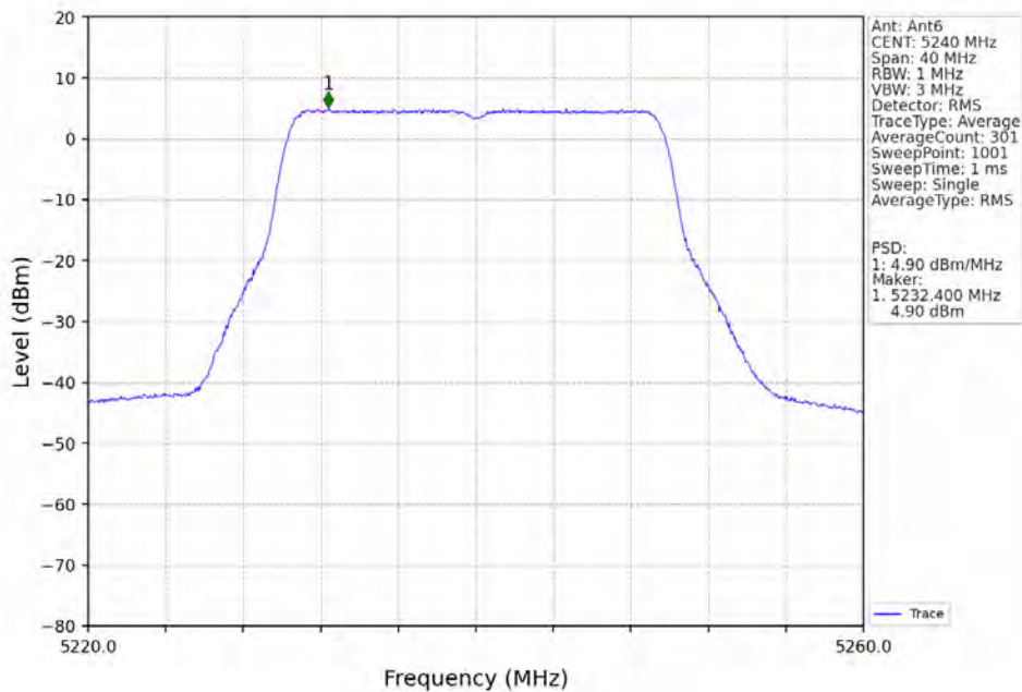
802.11be(EHT20)_HCH_5240MHz_RU242_Left_Ant6_NTNV
