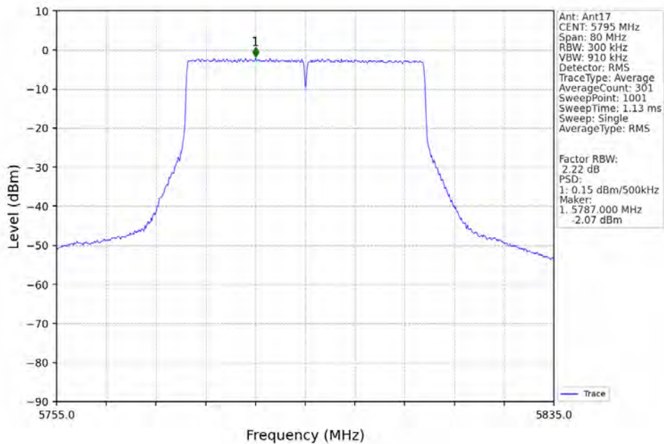
802.11be(EHT40)_HCH_5795MHz_RU484_Left_Ant17_NTNV
