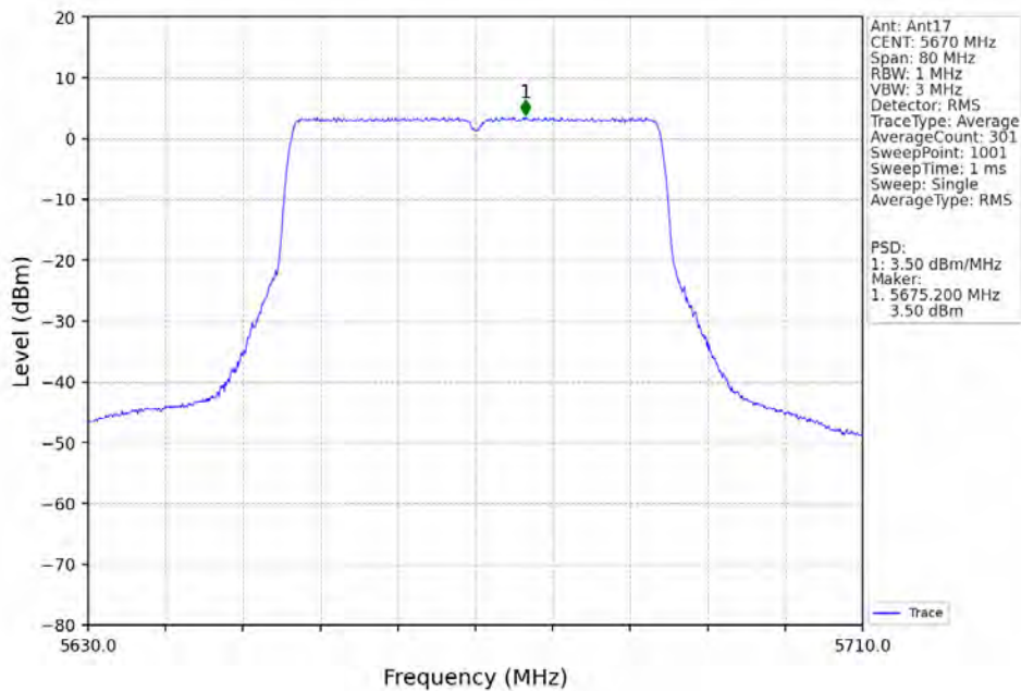
802.11be(EHT40)_HCH_5670MHz_RU484_Left_Ant17_NTNV
