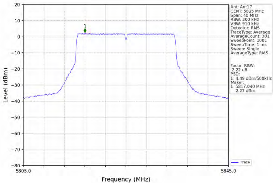
802.11ax(HEW20)_HCH_5825MHz_RU242_Left_Ant17_NTNV
