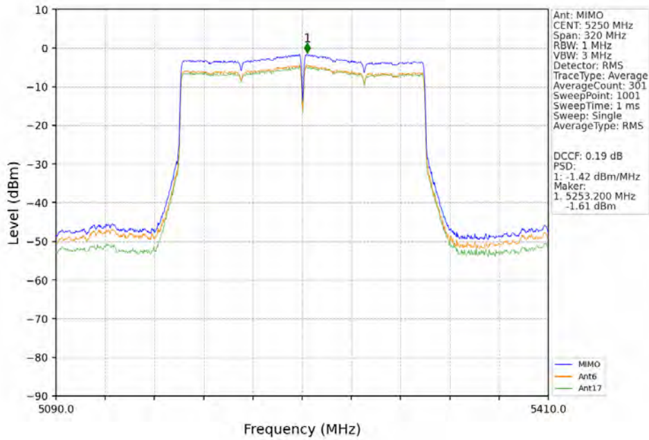
802.11be(EHT160)_MCH_5250MHz_2xRU996_Left_MIMO_NTNV
