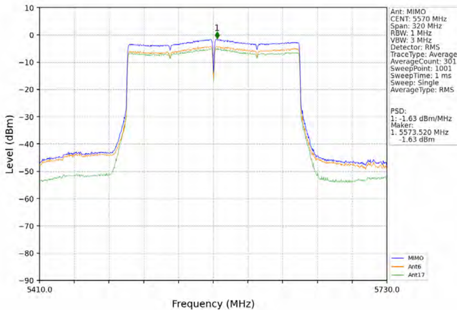
802.11be(EHT160)_MCH_5570MHz_2xRU996_Left_MIMO_NTNV
