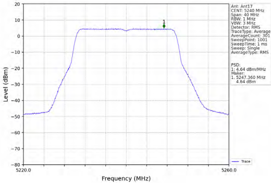
802.11be(EHT20)_HCH_5240MHz_RU242_Left_MIMO_NTNV
