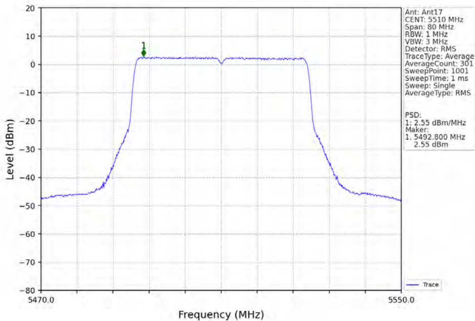
802.11be(EHT40)_LCH_5510MHz_RU484_Left_Ant17_NTNV
