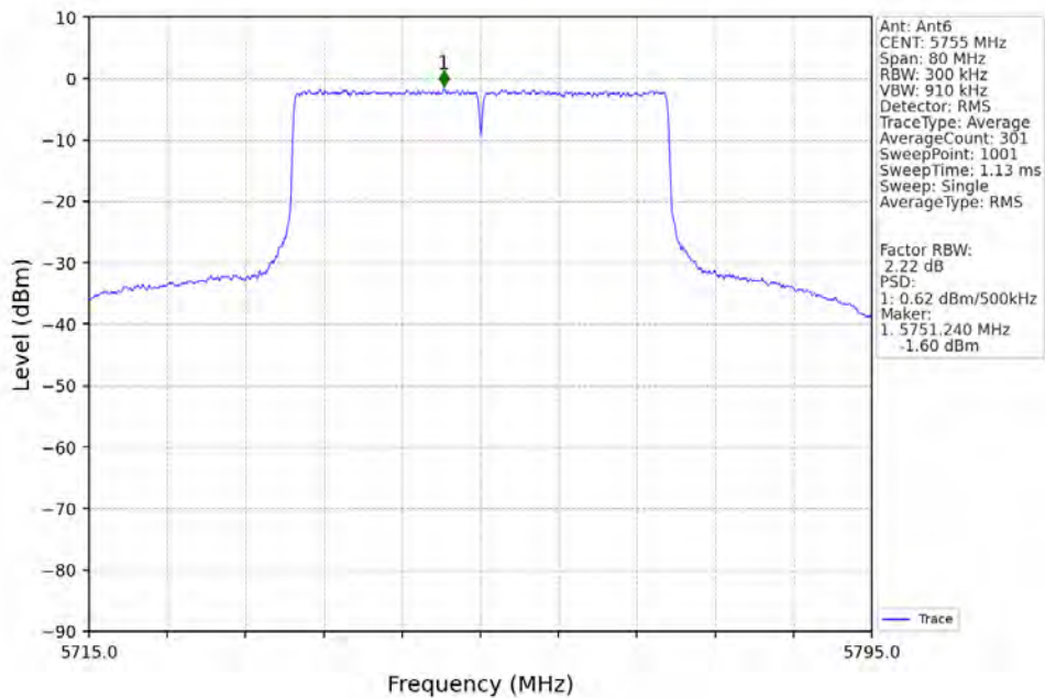
802.11ax(HEW40) LCH_5755MHz_RU484_Left_Ant6_NTNV
