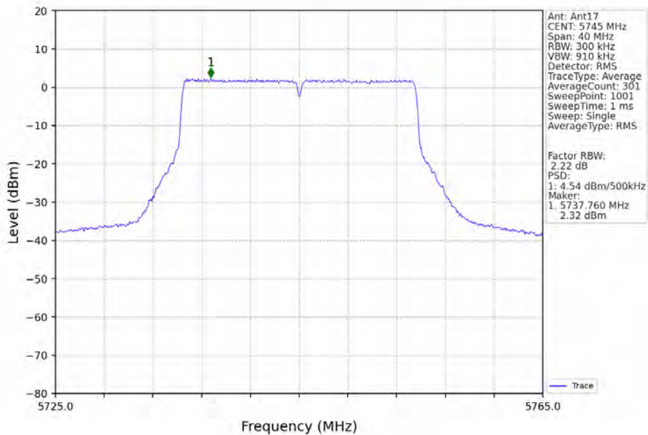
802.11be(EHT20)_LCH_5745MHz_RU242_Left_Ant17_NTNV
