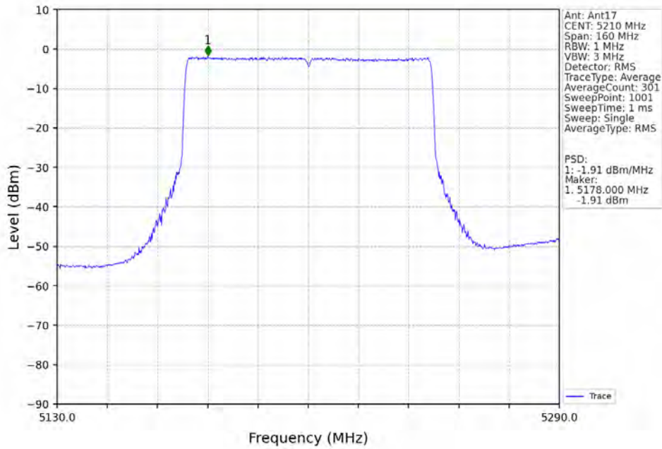
802.11be(EHT80)_MCH_5210MHz_RU996_Left_MIMO_NTNV
