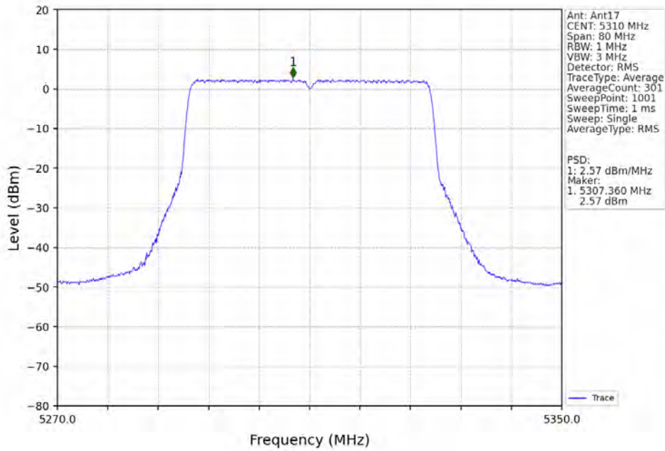
802.11be(EHT40)_HCH_5310MHz_RU484_Left_MIMO_NTNV
