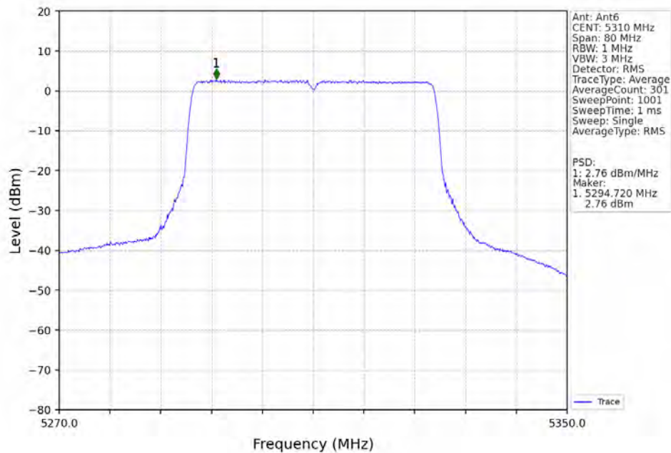
802.11be(EHT40)_HCH_5310MHz_RU484_Left_Ant6_NTNV
