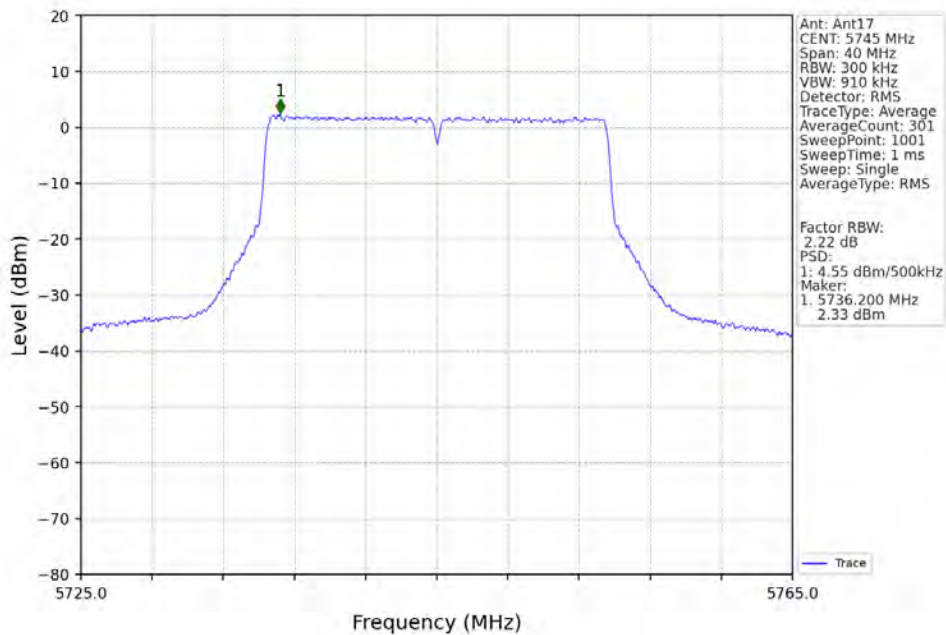
802.11ax(HEW20)_LCH_5745MHz_RU242_Left_Ant17_NTNV
