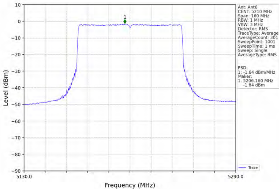
802.11be(EHT80)_MCH_5210MHz_RU996_Left_Ant6_NTNV
