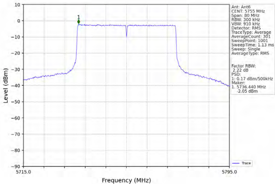
802.11be(EHT40)_LCH_5755MHz_RU484_Left_Ant6_NTNV
