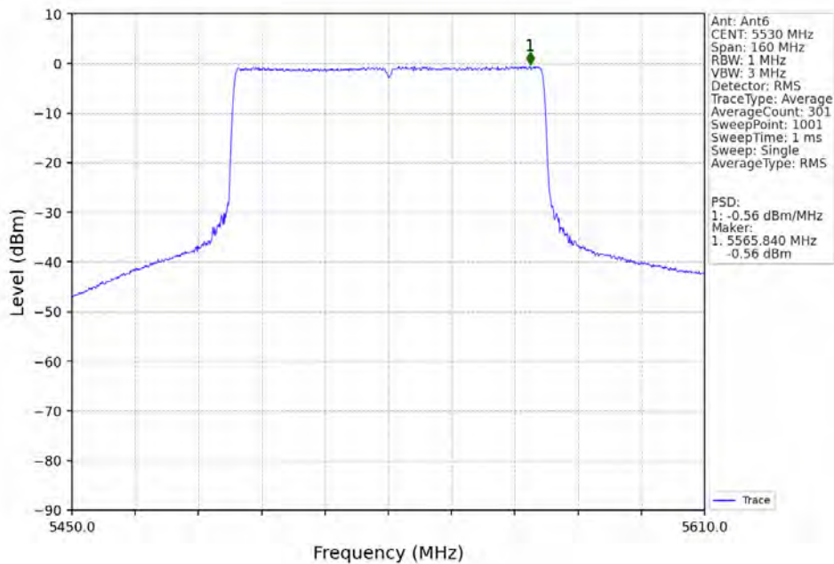
802.11be(EHT80)_LCH_5530MHz_RU996_Left_Ant6_NTNV
