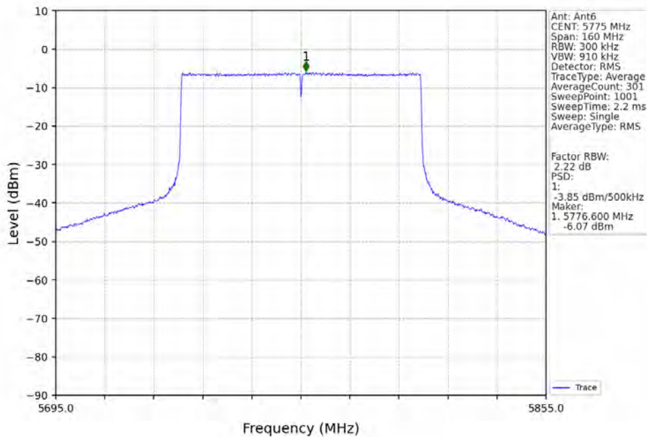
802.11ax(HEW80)_MCH_5775MHz_RU996_Left_Ant6_NTNV
