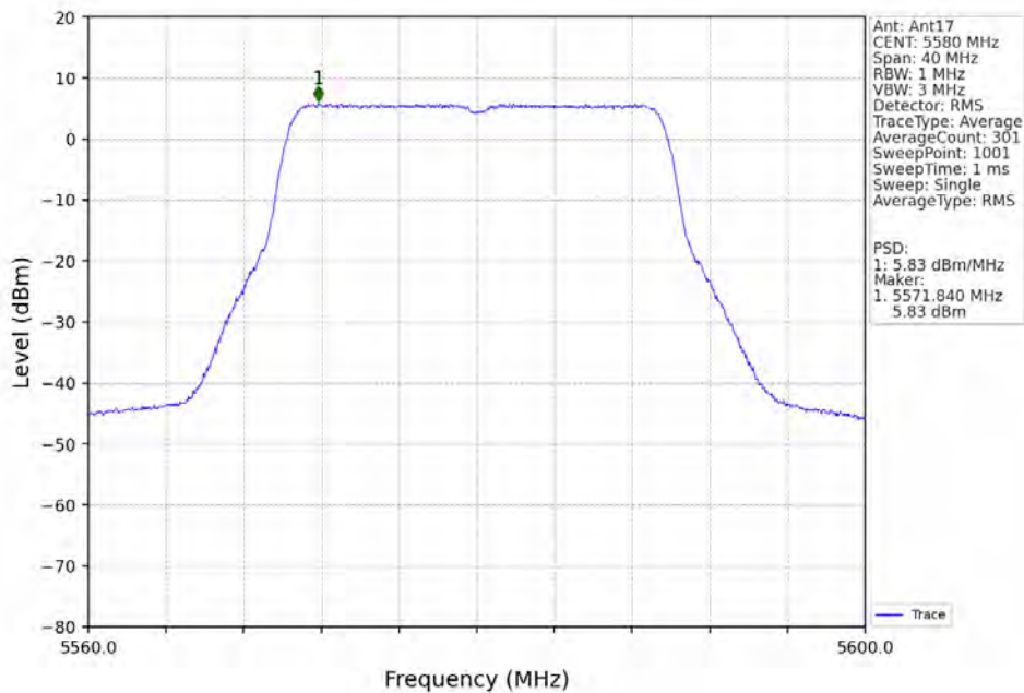
802.11be(EHT20)_MCH_5580MHz_RU242_Left_Ant17_NTNV
