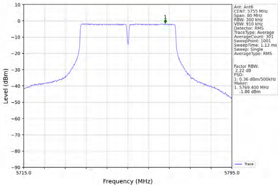
802.11ac(VHT40)_LCH_5755MHz_Ant6_NTNV
