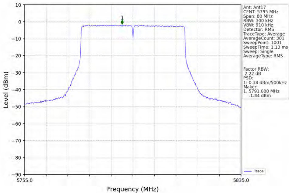
802.11ax(HEW40)_HCH_5795MHz_RU484_Left_Ant17_NTNV
