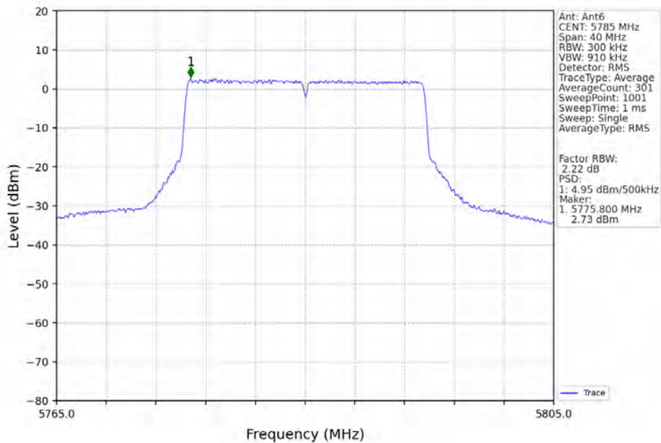
802.11be(EHT20)_MCH_5785MHz_RU242_Left_Ant6_NTNV
