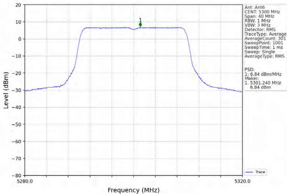
802.11be(EHT20)_MCH_5300MHz_RU242_Left_Ant6_NTNV
