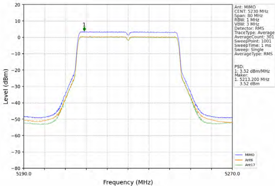
802.11be(EHT40)_HCH_5230MHz_RU484_Left_MIMO_NTNV
