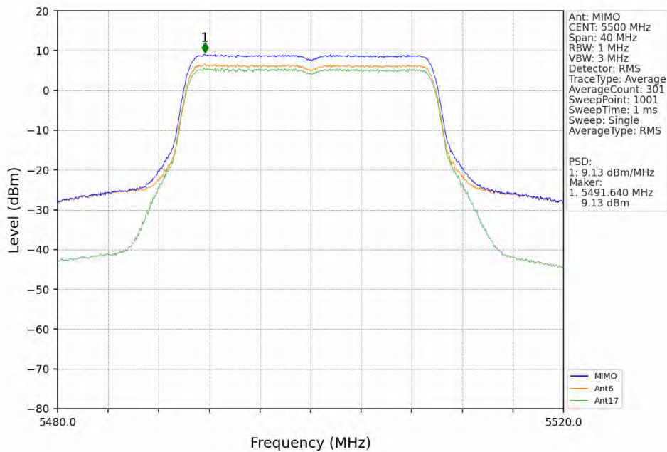
802.11be(EHT20)_LCH_5500MHz_RU242_Left_MIMO_NTNV
