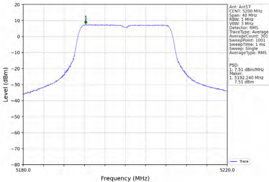
802.11n(HT20)_MCH_5200MHz_Ant17_NTNV
