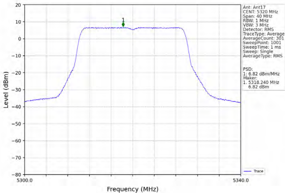
802.11ax(HEW20)_HCH_5320MHz_RU242_Left_Ant17_NTNV
