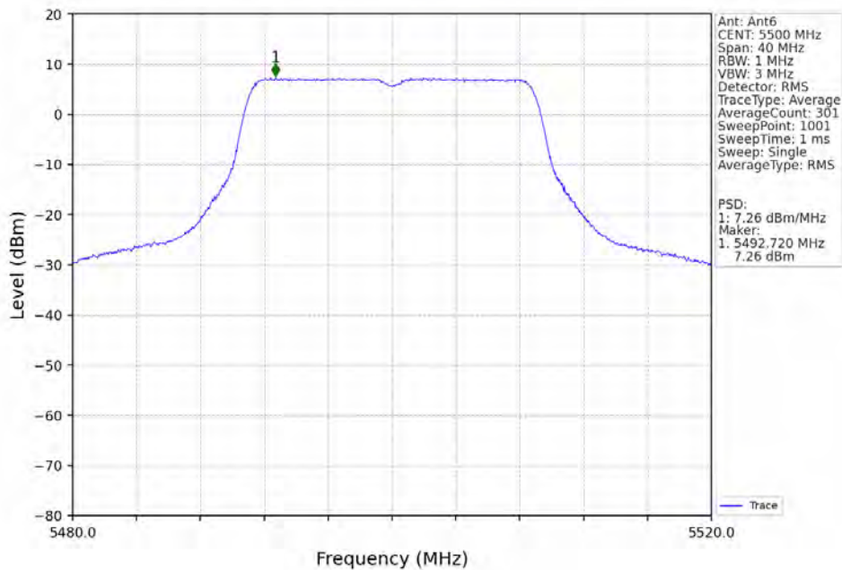
802.11ac(VHT20) LCH 5500MHz Ant6 NTN
