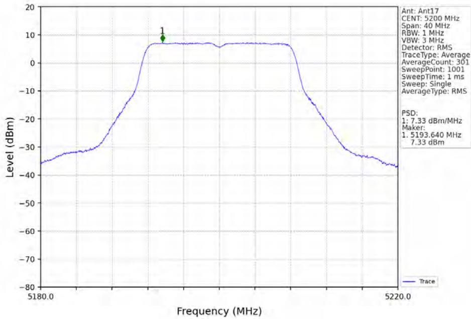
802.11a MCH 5200MHz MIMO NTN
