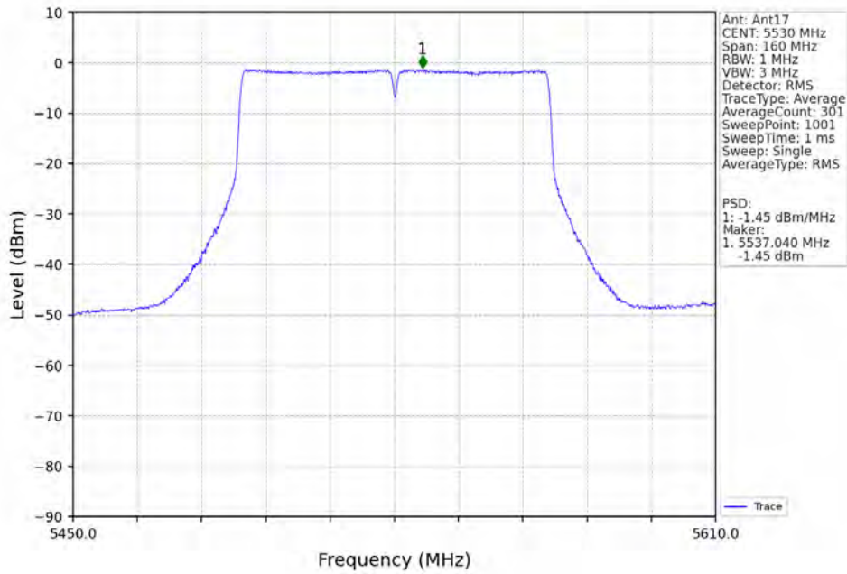
802.11ac(VHT80)_LCH_5530MHz MIMO NTN
