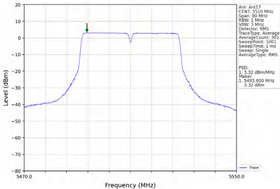
802.11n(HT40)_LCH_5510MHz_Ant17_NTNV
