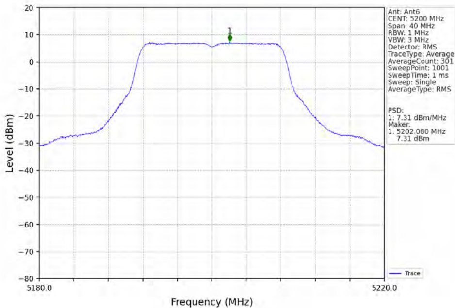
802.11a MCH 5200MHz Ant6 NTN
