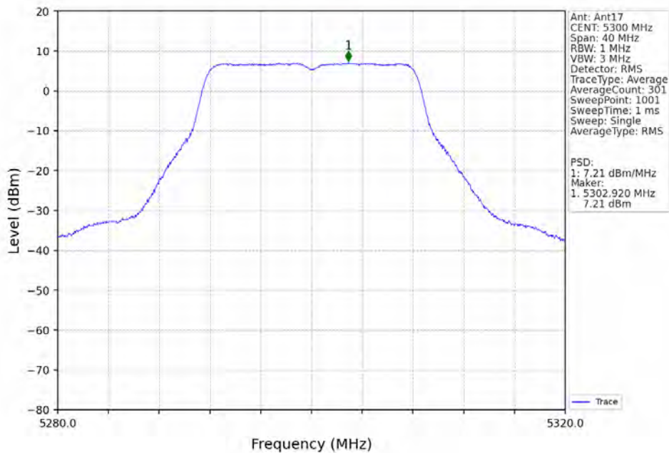
802.11a_MCH_5300MHz_Ant17_NTNV
