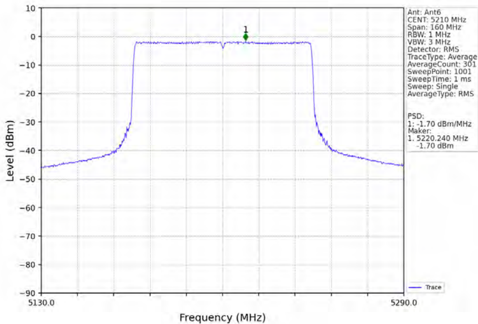
802.11ax(HEW80)_MCH_5210MHz_RU996_Left_Ant6_NTNV
