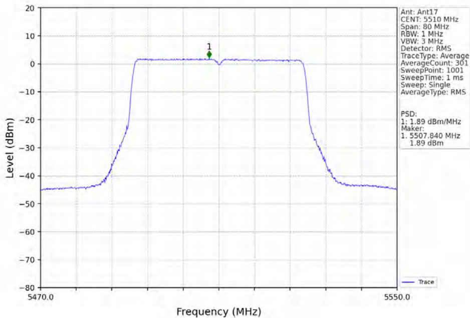
802.11ax(HEW40)_LCH_5510MHz_RU484_Left_Ant17_NTNV
