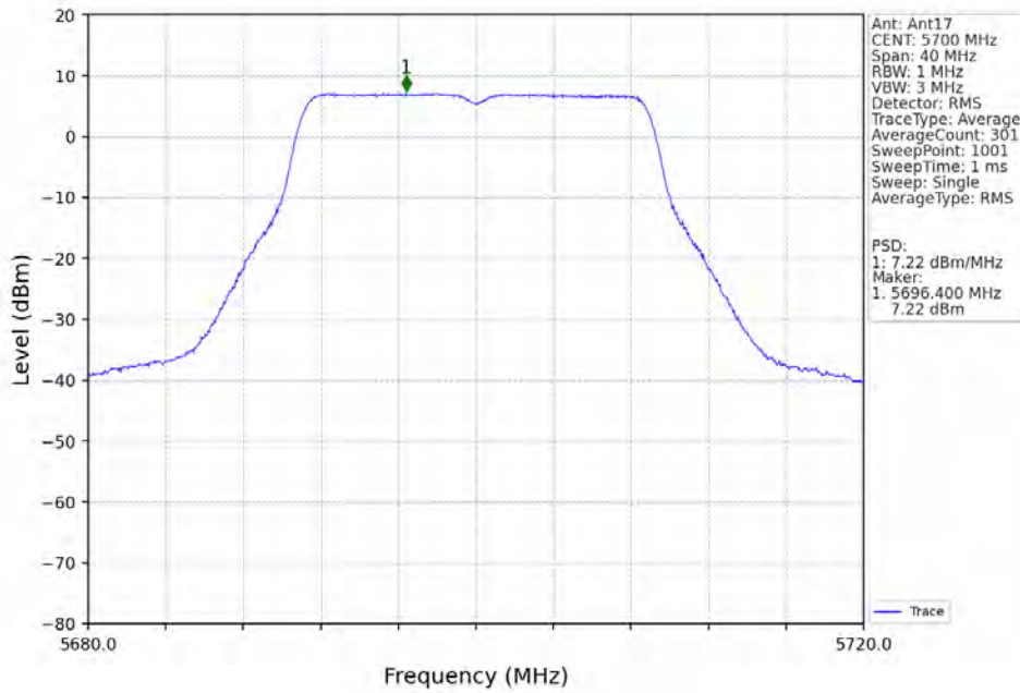
802.11ac(VHT20)_HCH_5700MHz MIMO NTN
