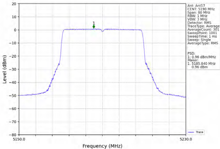
802.11ax(HEW40)_LCH_5190MHz_RU484_Left_Ant17_NTNV
