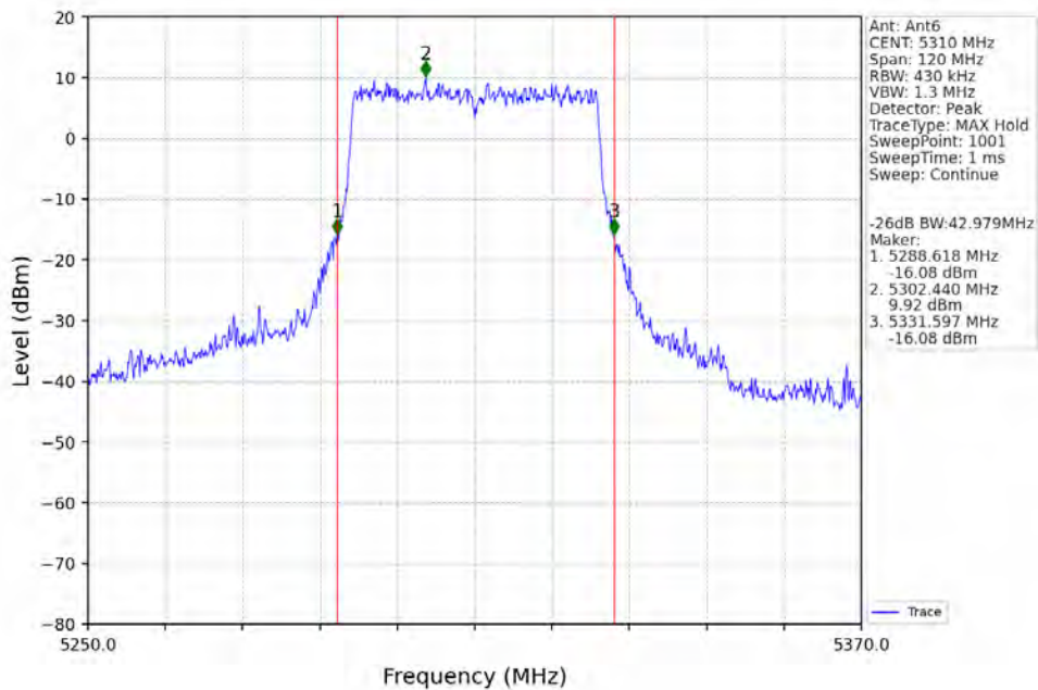
802.11be(EHT40)_HCH_5310MHz_RU484_Left_Ant6_NTNV
