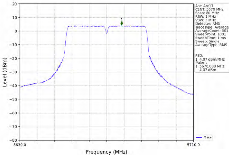
802.11n(HT40)_HCH_5670MHz_Ant17_NTNV
