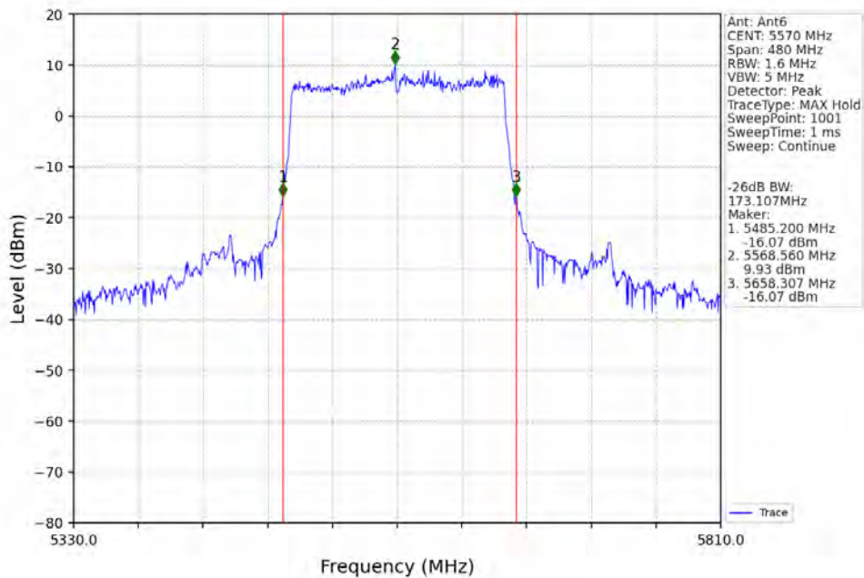
802.11be(EHT160) MCH 5570MHz 2xRU996 Left Ant6 NTN
