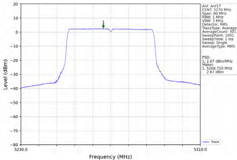
802.11ax(HEW40)_LCH_5270MHz_RU484_Left_Ant17_NTNV
