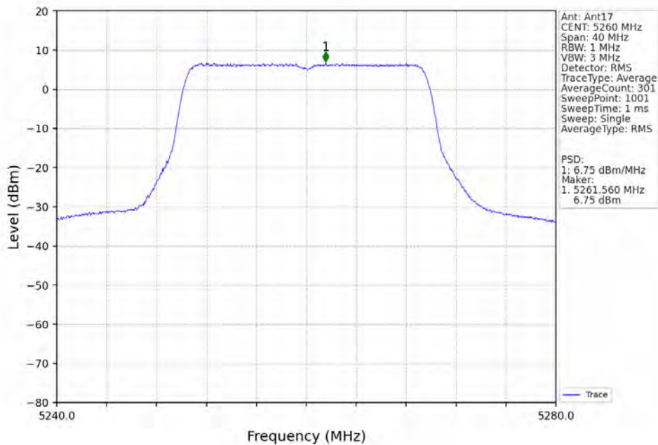
802.11ax(HEW20)_LCH_5260MHz_RU242_Left_Ant17_NTNV
