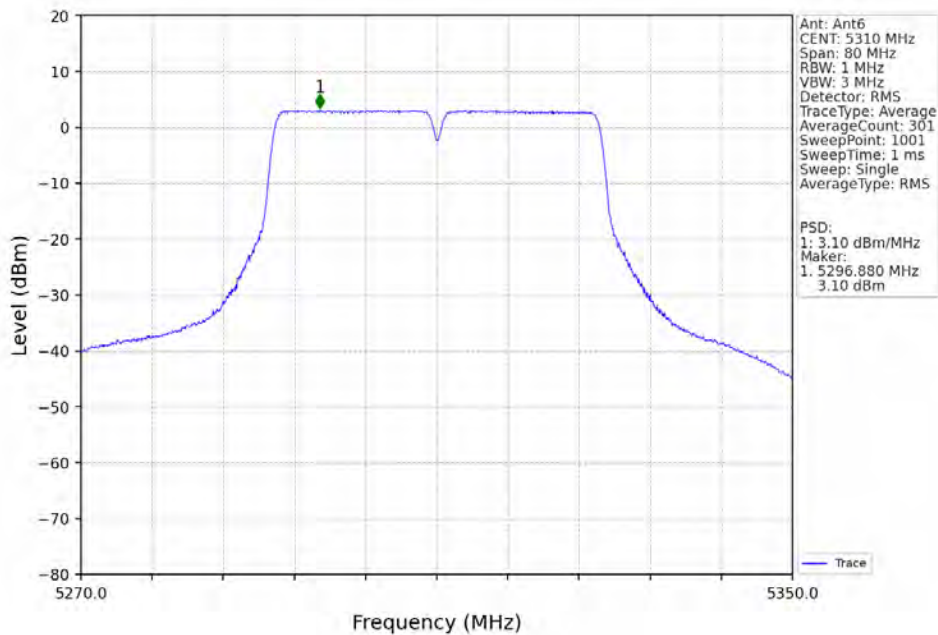
802.11ac(VHT40) HCH 5310MHz Ant6 NTN
