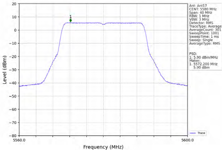
802.11ax(HEW20)_MCH_5580MHz_RU242_Left_Ant17_NTNV
