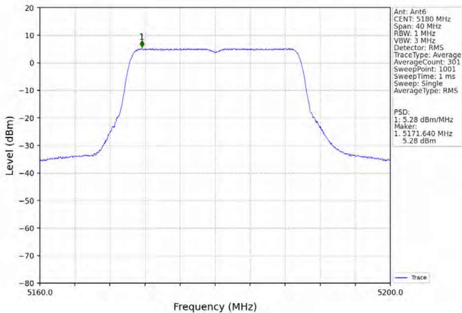
802.11be(EHT20)_LCH_5180MHz_RU242_Left_Ant6_NTNV
