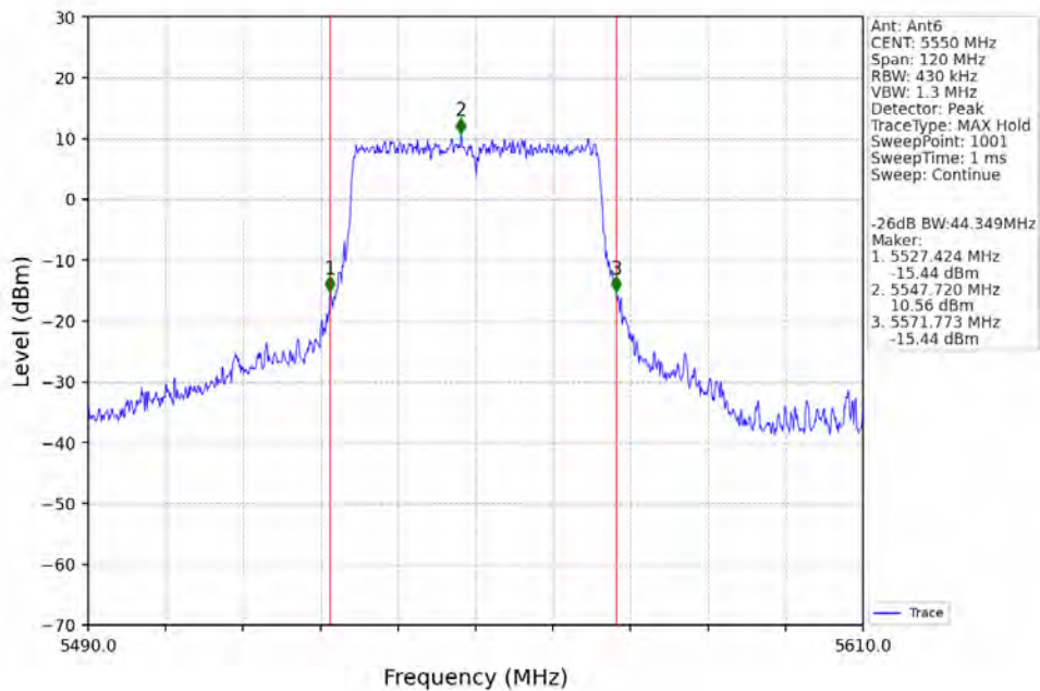
802.11be(EHT40)_MCH_5550MHz_RU484_Left_Ant6_NTNV
