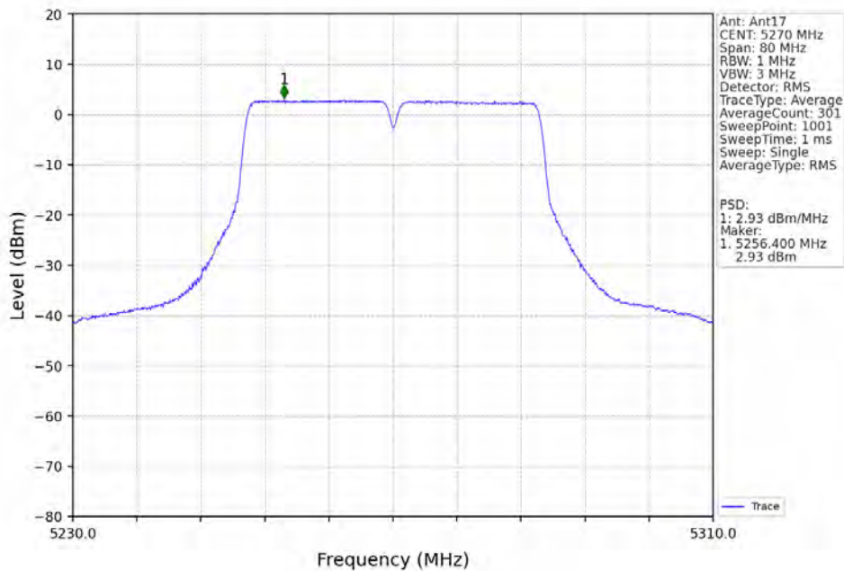
802.11ac(VHT40)_LCH_5270MHz_Ant17_NTNV
