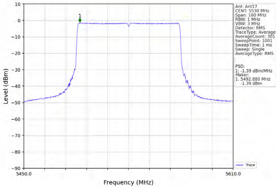
802.11ax(HEW80)_LCH_5530MHz_RU996_Left MIMO NTN
