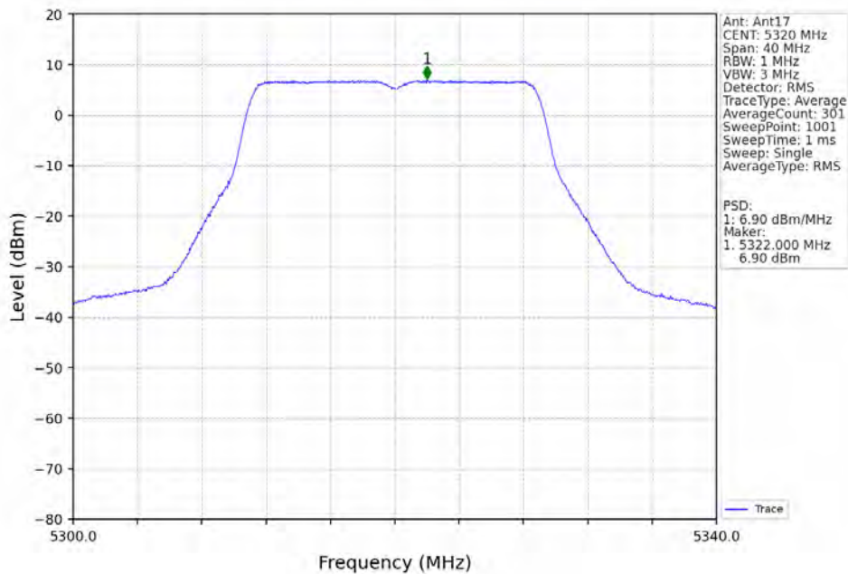
802.11ac(VHT20)_HCH_5320MHz_Ant17_NTNV
