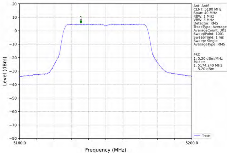
802.11ax(HEW20) LCH 5180MHz RU242 Left Ant6 NTN
