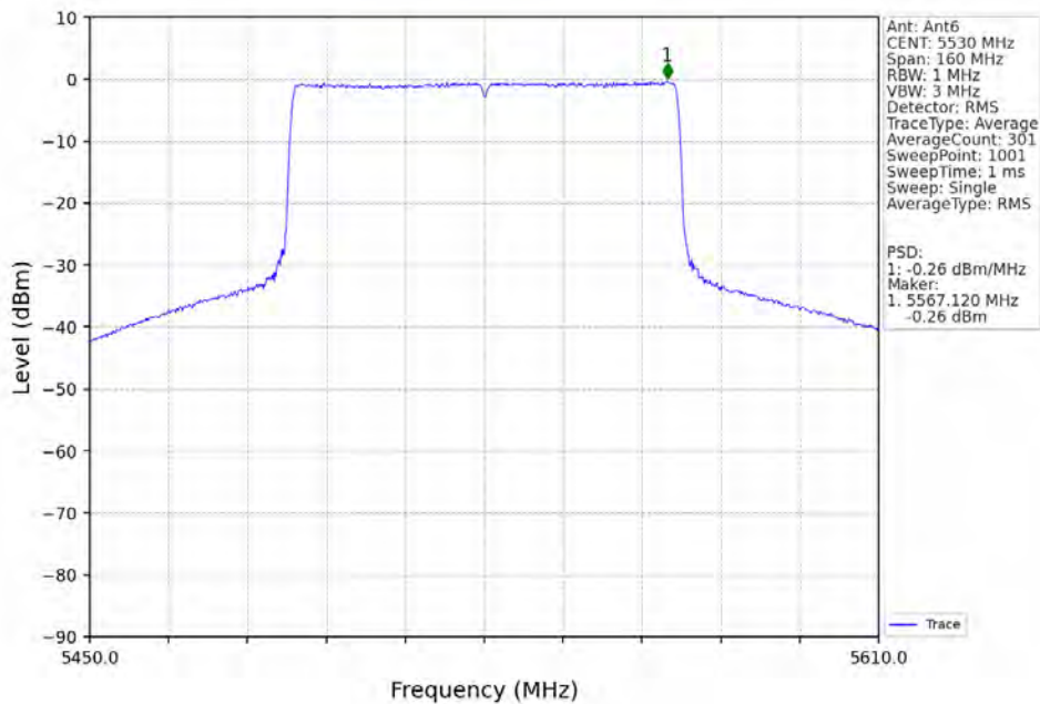
802.11ax(HEW80) LCH 5530MHz RU996 Left Ant6 NTN
