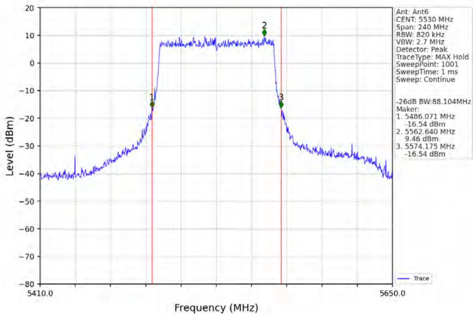
802.11be(EHT80)_LCH_5530MHz_RU996_Left_Ant6_NTNV
