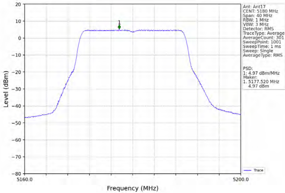
802.11be(EHT20)_LCH_5180MHz_RU242_Left_MIMO_NTNV
