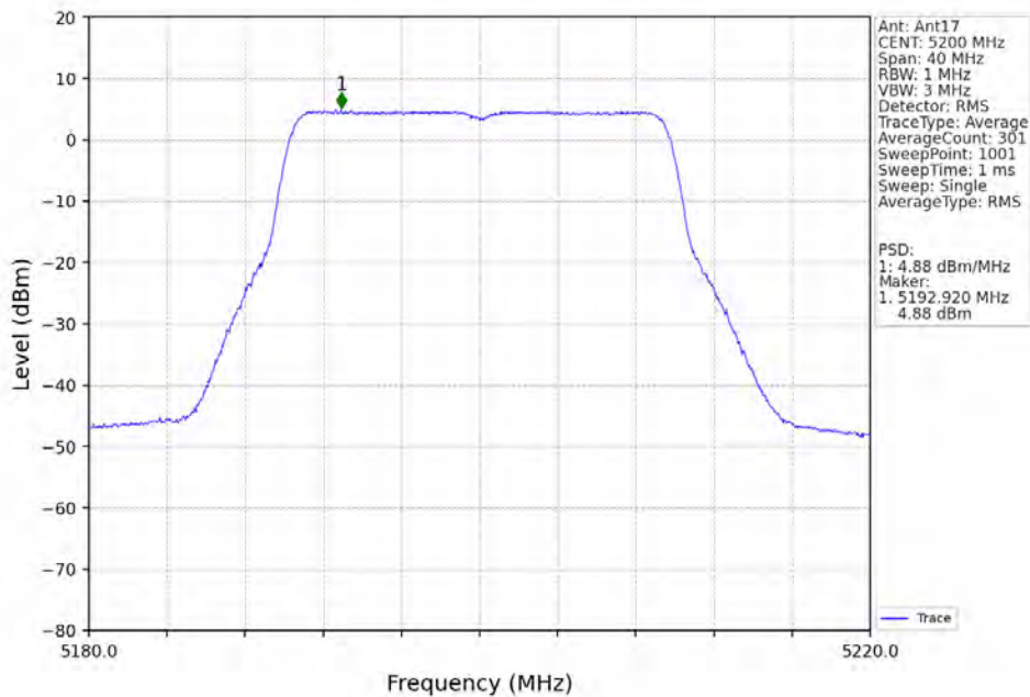
802.11ax(HEW20)_MCH_5200MHz_RU242_Left_Ant17_NTNV
