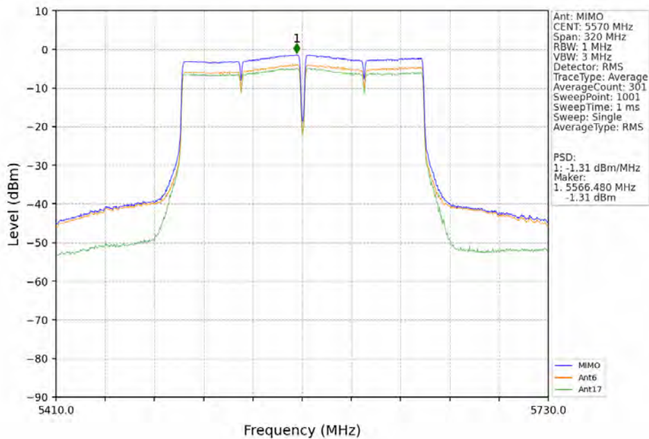
802.11ac(VHT160) MCH 5570MHz MIMO NTN
