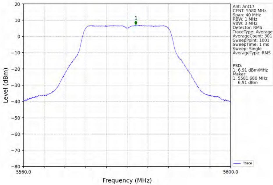
802.11a MCH 5580MHz MIMO NTN
