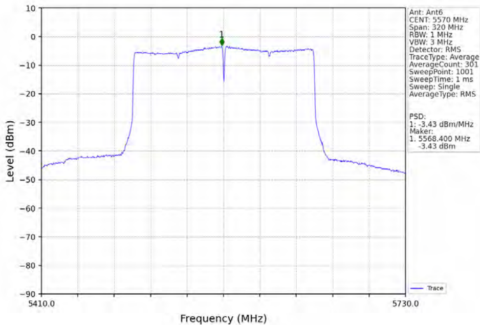
802.11ax(HEW160)_MCH_5570MHz_2xRU996_Left_Ant6_NTNV
