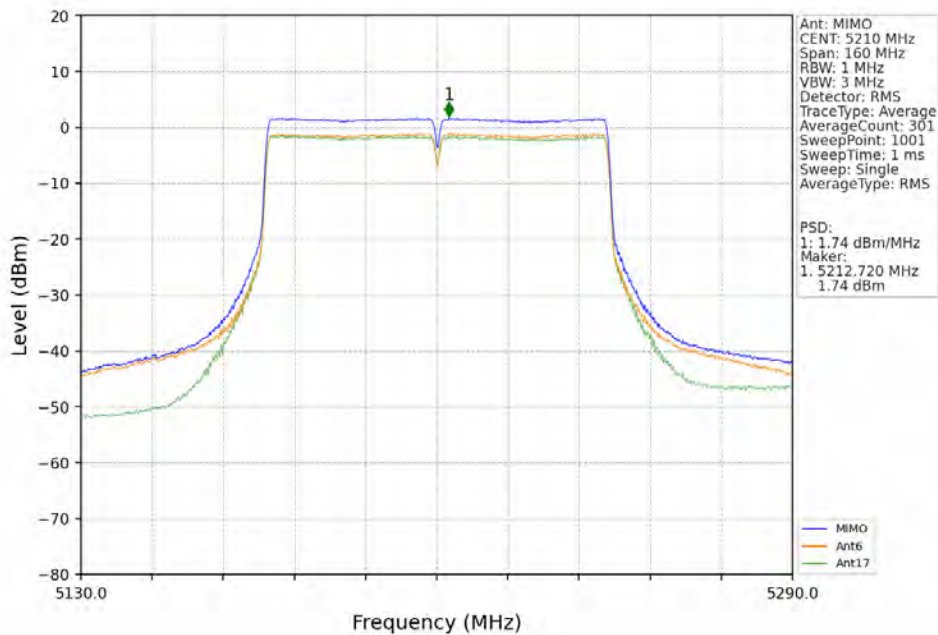
802.11ac(VHT80)_MCH_5210MHz MIMO NTN
