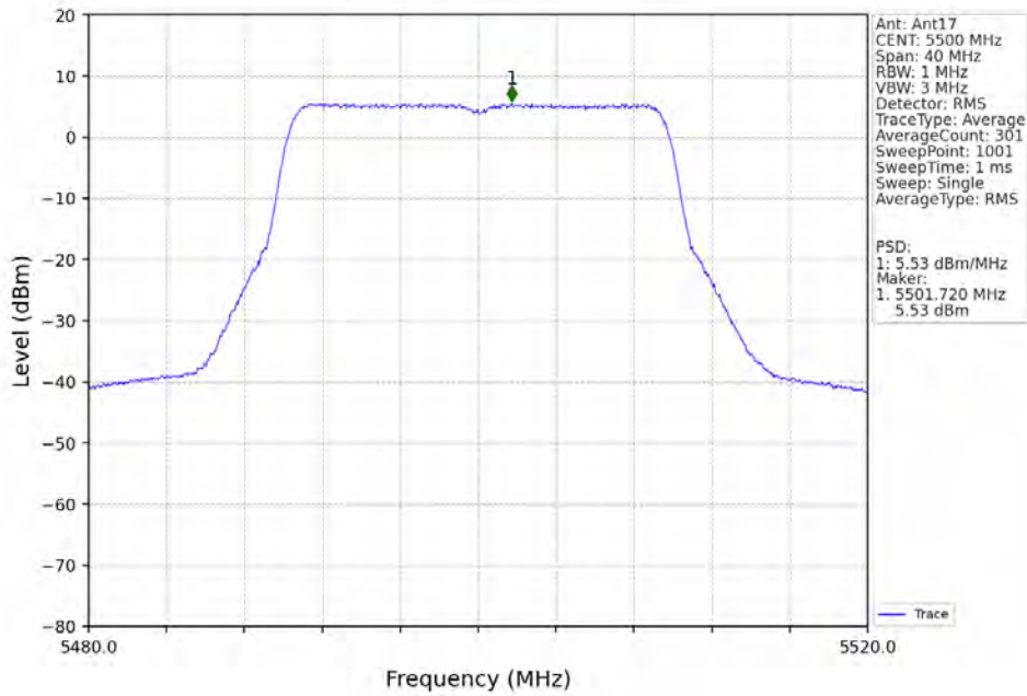
802.11ax(HEW20)_LCH_5500MHz_RU242_Left MIMO NTN
