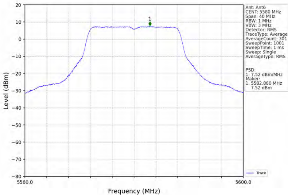
802.11a MCH 5580MHz Ant6 NTN
