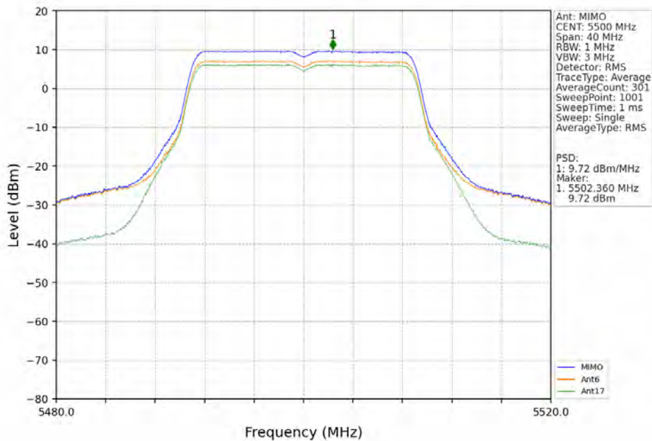
802.11ac(VHT20)_LCH_5500MHz MIMO NTN
