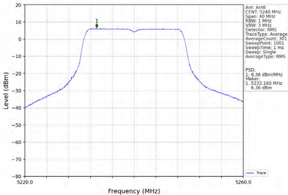
802.11n(HT20) HCH 5240MHz Ant6 NTN
