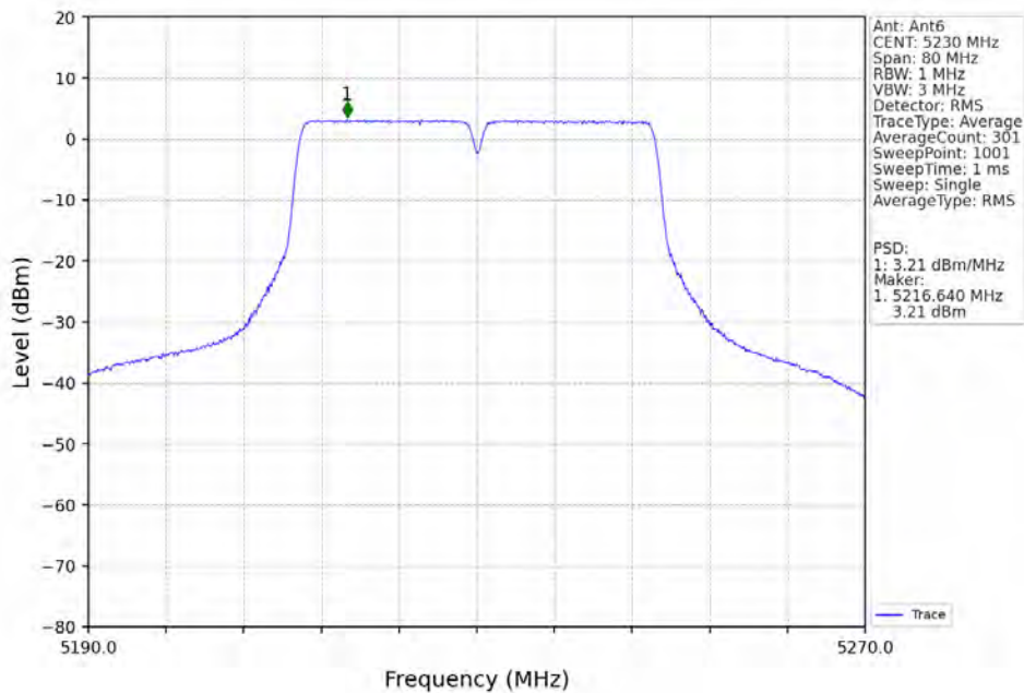
802.11ac(VHT40) HCH 5230MHz Ant6 NTN
