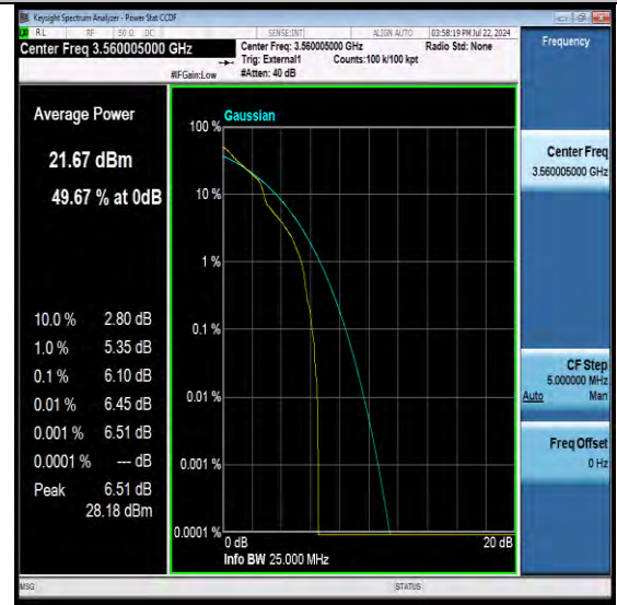
NTNV-N48-PC3-30-20-L-DFT-QPSK-Edge_1RB_Left-PASS
