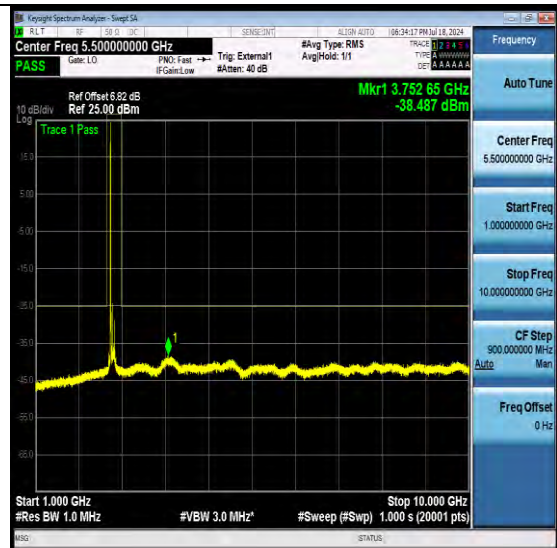
NTNV-N41-PC3-30-80-M-DFT-QPSK-Edge_1RB_Left-Ant1-PASS
