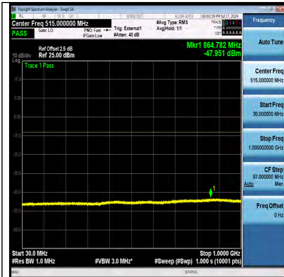
NTNV-N77-3450-3550-PC2-30-60-L-DFT-QPSK-E dge 1RB Left-Ant1-PASS
