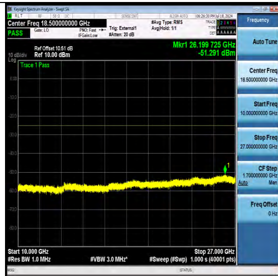
NTNV-N41-PC3-30-60-M-DFT-QPSK-Edge_1RB_Left-Ant1-PASS
