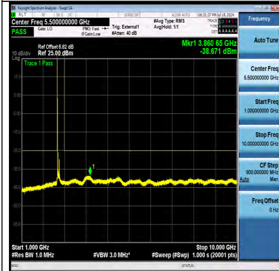
NTN-N41-PC3-30-80-L-DFT-QPSK-Edge_1RB_Left-Ant1-PASS
