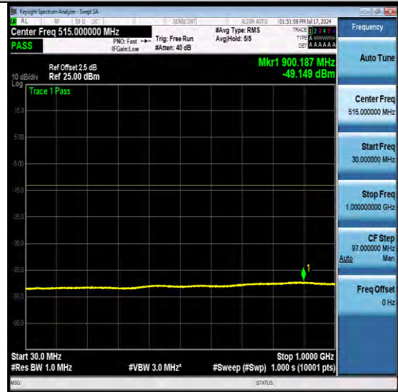
NTNV-N66-PC3-15-5-H-DFT-QPSK-Edge_1RB_L eft-Ant1-PASS
