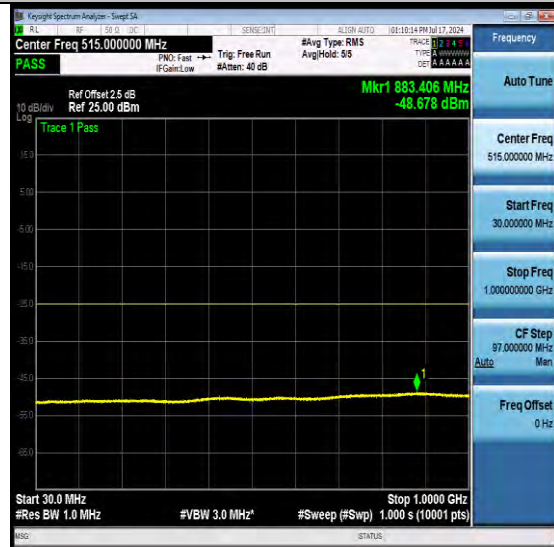
NTN-N7-PC3-15-50-M-DFT-QPSK-Edge_1RB_L eft-Ant1-PASS
