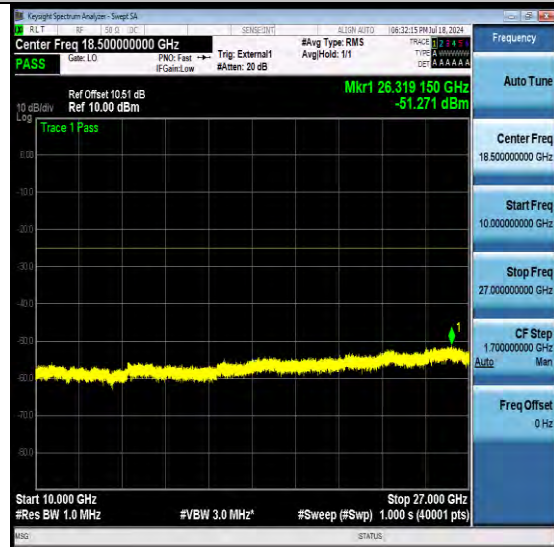
NTN-N41-PC3-30-80-L-DFT-QPSK-Edge_1RB_Left-Ant1-PASS
