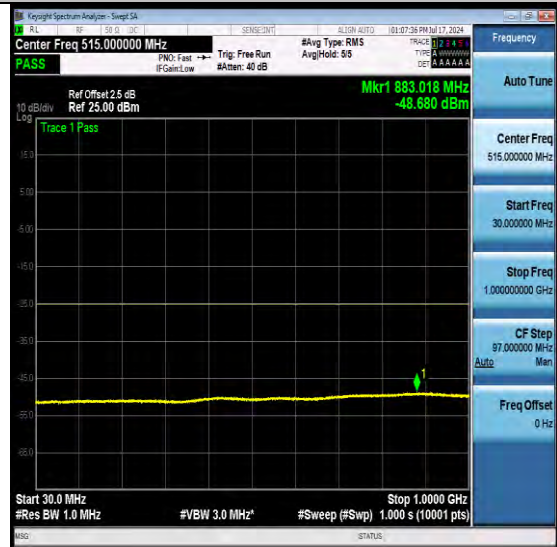
NTNV-N7-PC3-15-25-H-DFT-QPSK-Edge_1RB_L eft-Ant1-PASS
