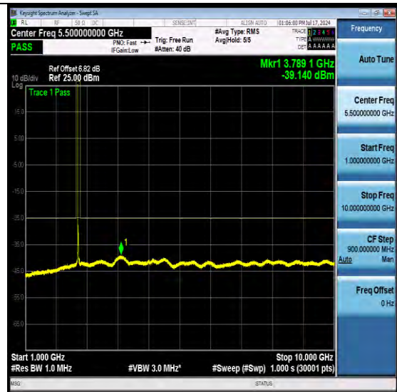
NTNV-N7-PC3-15-25-M-DFT-QPSK-Edge_1RB_L eft-Ant1-PASS
