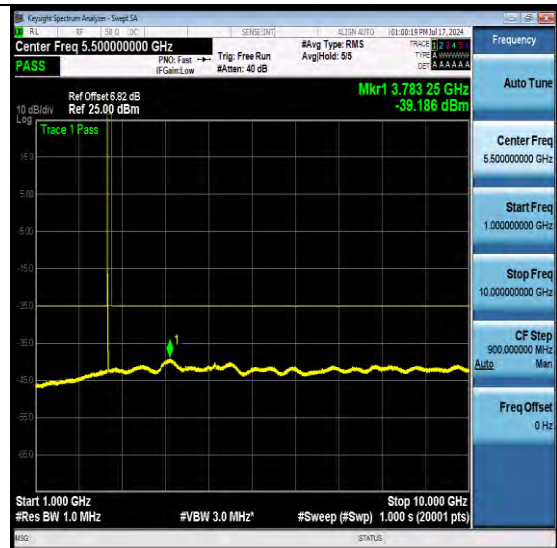
NTNV-N7-PC3-15-5-L-DFT-QPSK-Edge_1RB_Lef t-Ant1-PASS
