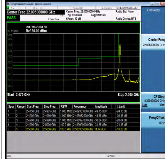
NTNV-N7-PC3-15-5-L-DFT-QPSK-Edge_1RB_Lef t-Ant1-PASS
