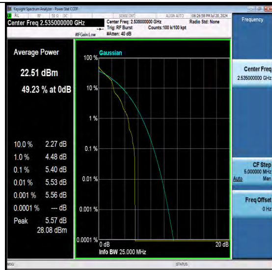
NTNV-N7-PC3-15-20-M-DFT-QPSK-Edge_1RB_L eft-PASS
