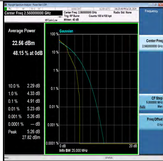
NTNV-N7-PC3-15-20-H-DFT-QPSK-Edge_1RB_L eft-PASS
