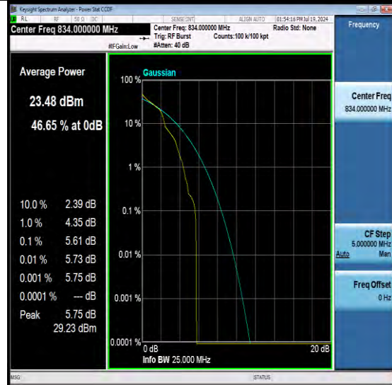
NTNV-N26-824-849-PC3-15-20-L-DFT-QPSK-Edge 1RB Left-PASS
