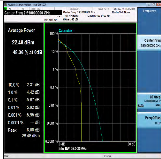
NTNV-N7-PC3-15-20-L-DFT-QPSK-Edge_1RB_Left-PASS
