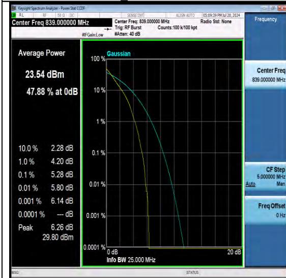
NTNV-N26-824-849-PC3-15-20-H-DFT-QPSK-Out er Full-PASS
