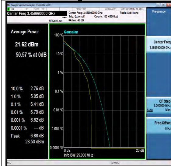
NTNV-N77-3450-3550-PC2-30-20-L-DFT-QPSK-Edge 1RB Left-PASS
