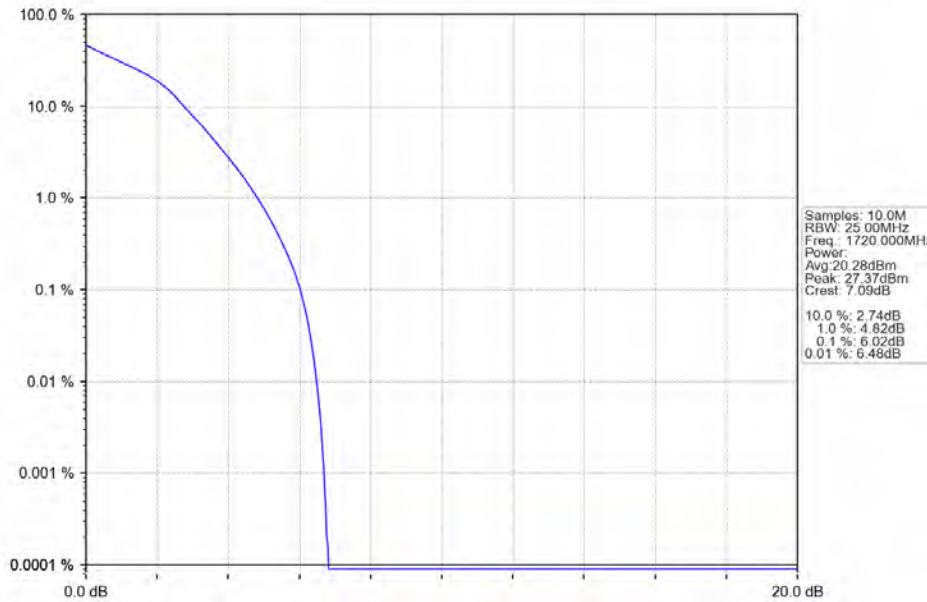
Band66_20MHz_16QAM_LCH_1720MHz_RB_100_0_NTNV
