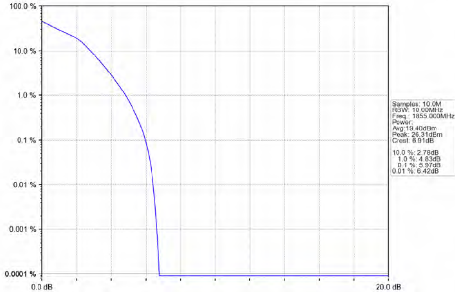
Band2_10MHz_16QAM_LCH_1855MHz_RB_50_0_NTNV
