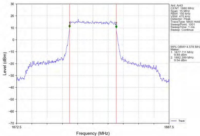
Band2_5MHz_QPSK_MCH_1880MHz_RB_25_0_NTNV
